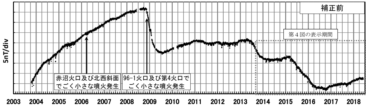
第5図 ポンマチ南東と女満別観測施設の全磁力日平均値差 (2003年10月16日～2018年6月4日) 年周変化補正と太陽活動等によるノイズ補正を行っていない。
