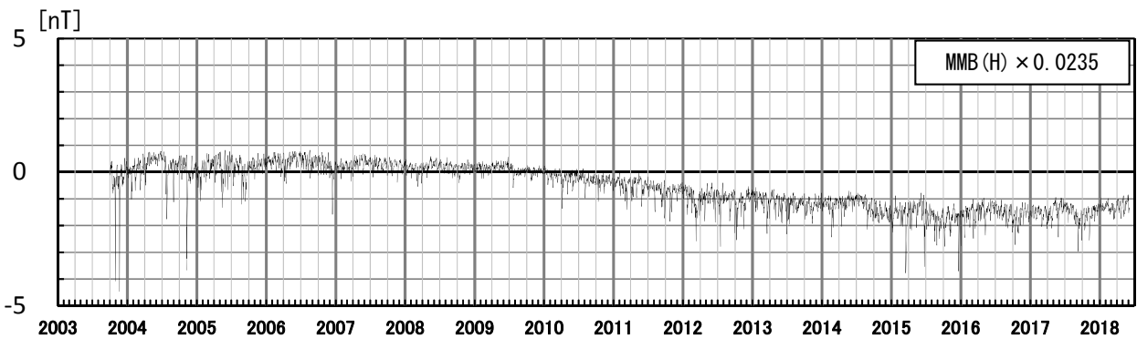
第7図 女満別観測施設の地磁気水平成分から求めた太陽活動等によるノイズ量 (2003年10月16日～2018年6月4日)
