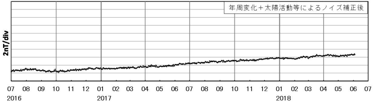
第3図 ポンマチ南東と女満別観測施設の全磁力日平均値差 (2016年7月1日~2018年6月4日) 年周変化補正と太陽活動等によるノイズ補正を行っている。
