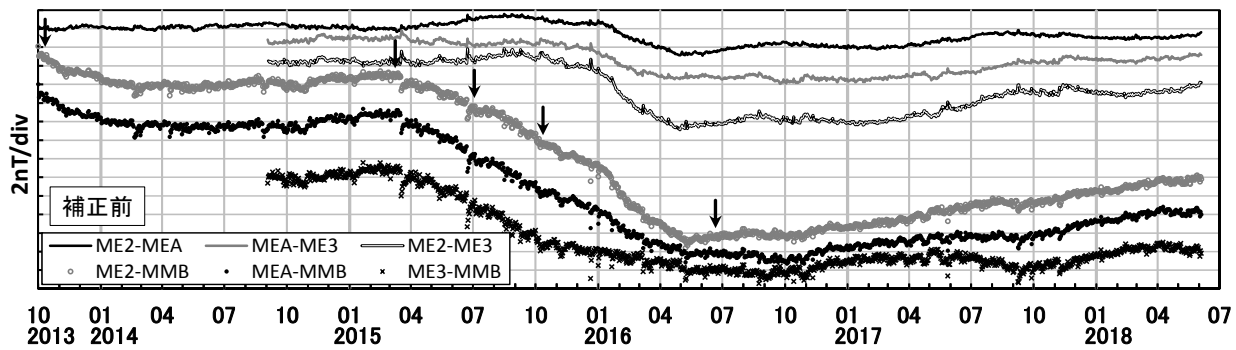
第4図 各連続観測点 (MEA、ME2、ME3) と女満別観測施設 (MMB) の全磁力日平均値差及び各連続観測点間の全磁力日平均値差 (2013年10月1日~2018年6月4日) 年周変化補正と太陽活動等によるノイズ補正を行っていない。図中の矢印は火山性微動の発生日を示す。
