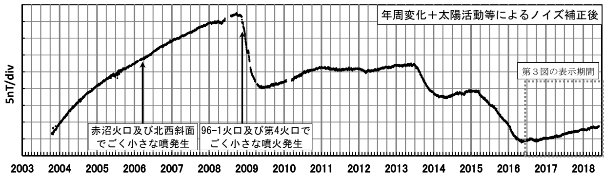
第2図 ポンマチ南東と女満別観測施設の全磁力日平均値差 (2003年10月16日～2018年6月4日) 年周変化補正と太陽活動等によるノイズ補正を行っている。
