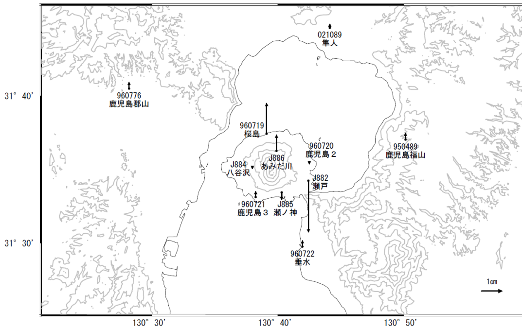
第 3-3 図 桜島周辺の電子基準点・気象庁 GNSS 観測点の統合解析による上下変動ベクトル図 (上段:2017年10月~2018年1月、下段:2016年12月~2018年1月)
