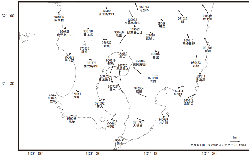
第3-1図 南九州地方におけるGNSS観測点の水平変動ベクトル図
