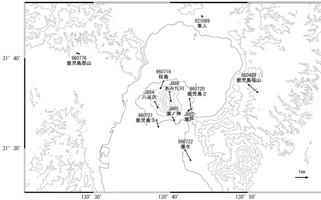
第3-2図 桜島周辺の電子基準点・気象庁GNSS観測点の統合解析による水平変動ベクトル図 (上段:2017年10月~2018年1月、下段:2016年12月~2018年1月)
