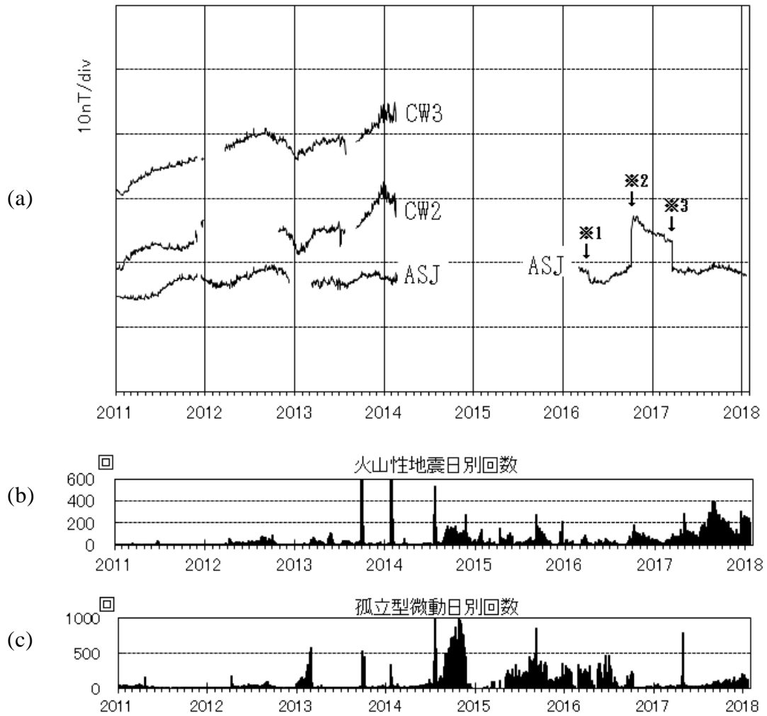
第2図 2011年1月から2018年1月まで連続観測点CW2、CW3、ASJにおける全磁力日平均値と参照点AHKの日平均値との差(a)、火山性地震日別回数(b)、孤立型微動日別回数(c)
