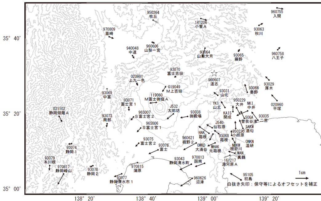
第3図 富士山周辺の電子基準点・気象庁・神奈川県温泉地学研究所 GNSS 観測点の統合解析による水平変動ベクトル図 (上段:2017年9月~2018年1月、下段:2016年12月~2018年1月)
