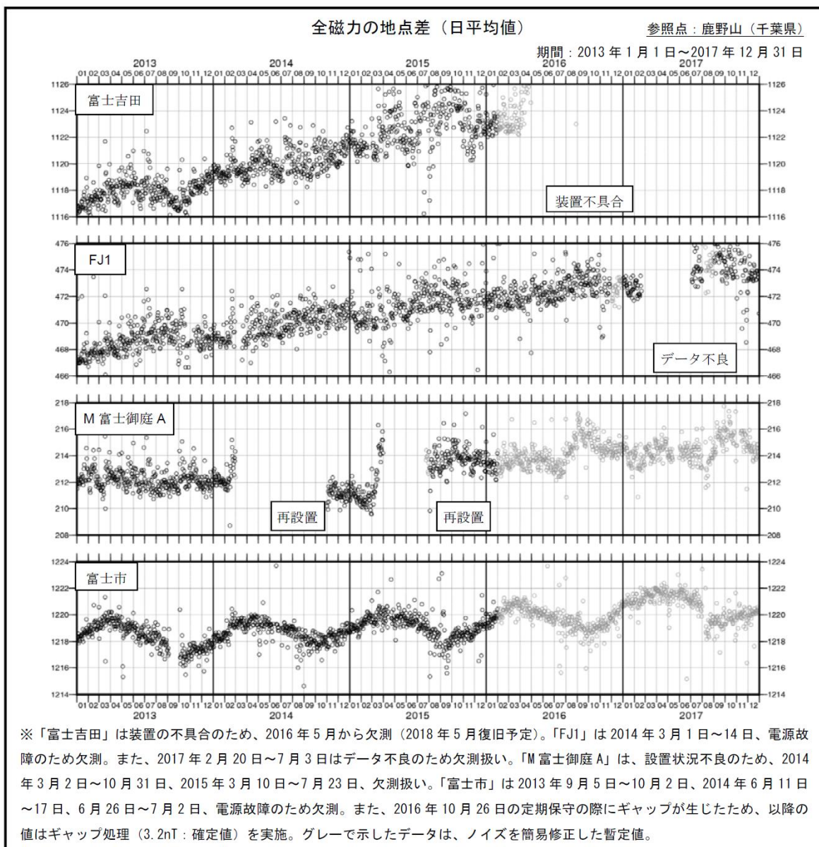
第5図 富士山における全磁力連続観測結果
