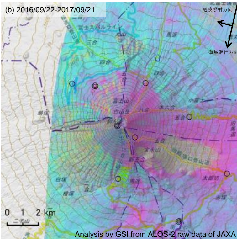
第4図 「だいち2号」PALSAR-2による富士山の解析結果
