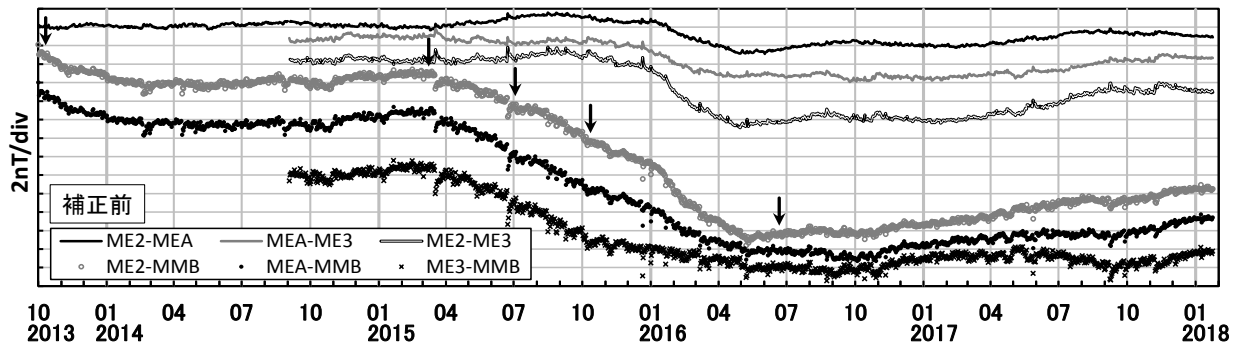
第4図 各連続観測点 (MEA、ME2、ME3) と女満別観測施設 (MMB) の全磁力日平均値差及び各連続観測点間の全磁力日平均値差 (2013年10月1日～2018年1月24日) 年周変化補正と太陽活動等によるノイズ補正を行っていない。図中の矢印は火山性微動の発生日を示す。
