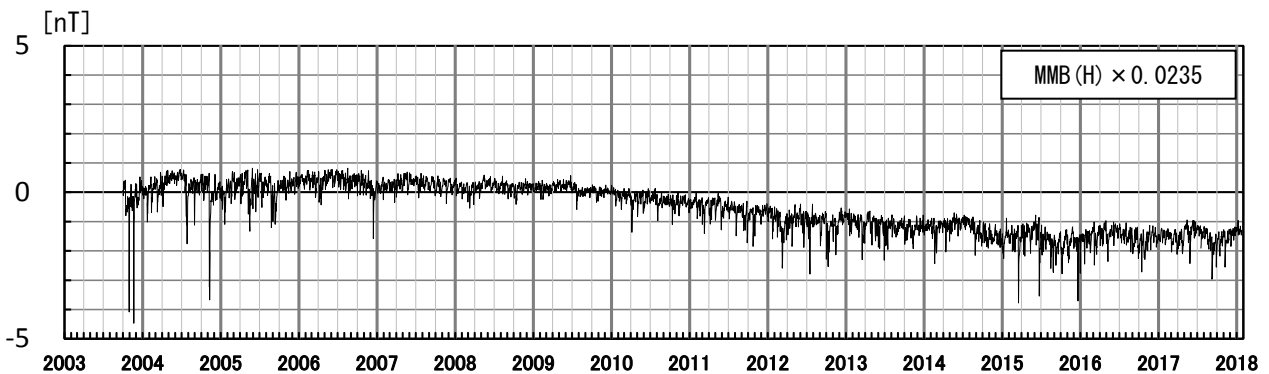
第7図 女満別観測施設の地磁気水平成分から求めた太陽活動等によるノイズ量 (2003年10月16日～2018年1月24日)
