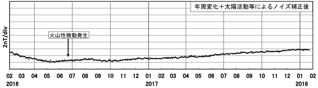
第3図 ポンマチ南東と女満別観測施設の全磁力日平均値差 (2016年2月1日～2018年1月24日) 年周変化補正と太陽活動等によるノイズ補正を行っている。
