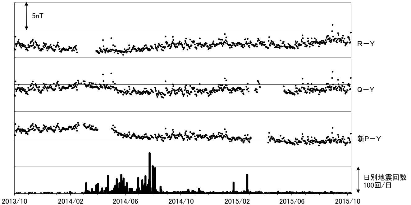
第3図 全磁力連続観測による全磁力値の変化及び日別地震回数（2013年10月～2015年10月8日）。連続観測点新P、QおよびRにおける八ヶ岳地球電磁気観測所（東京大学地震研究所）（Y）との全磁力の日平均値差。最下段に草津白根山で観測された日別地震回数を示す。
