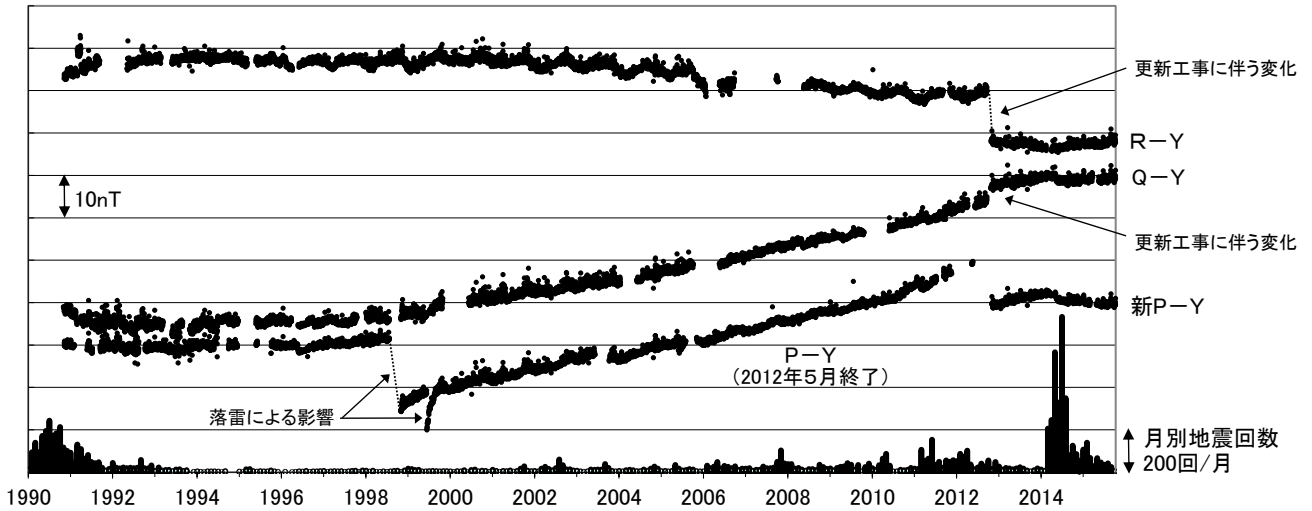
第2図 全磁力連続観測による全磁力値の変化及び月別地震回数（1990年1月～2015年10月8日）。連続観測点P、Q、Rおよび新Pにおける八ヶ岳地球電磁気観測所（東京大学地震研究所）（Y）との全磁力の日平均値差。最下段に草津白根山で観測された月別地震回数を示す。
