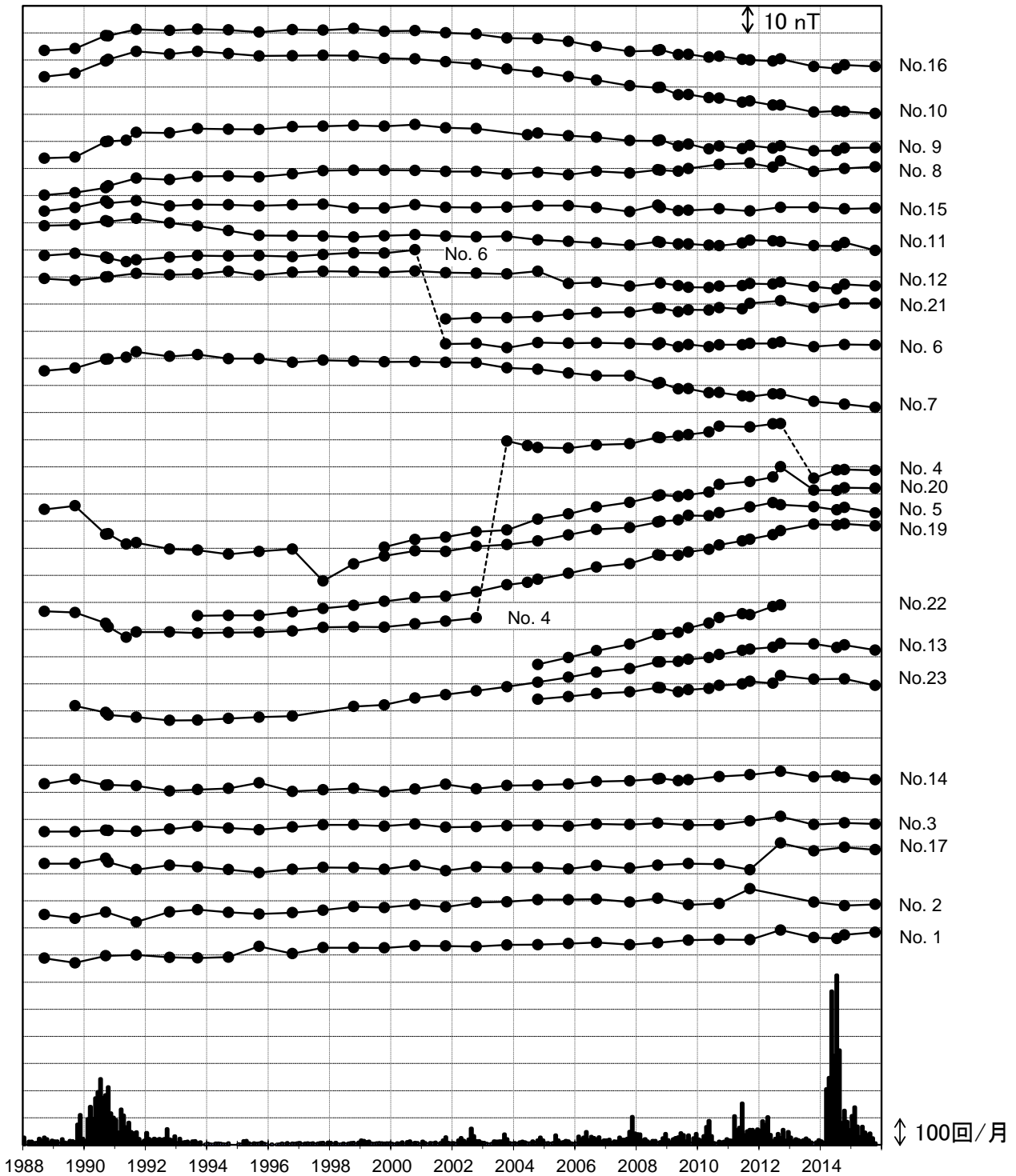
第4図 全磁力繰り返し観測による全磁力値の変化 (1988年9月～2015年10月)
