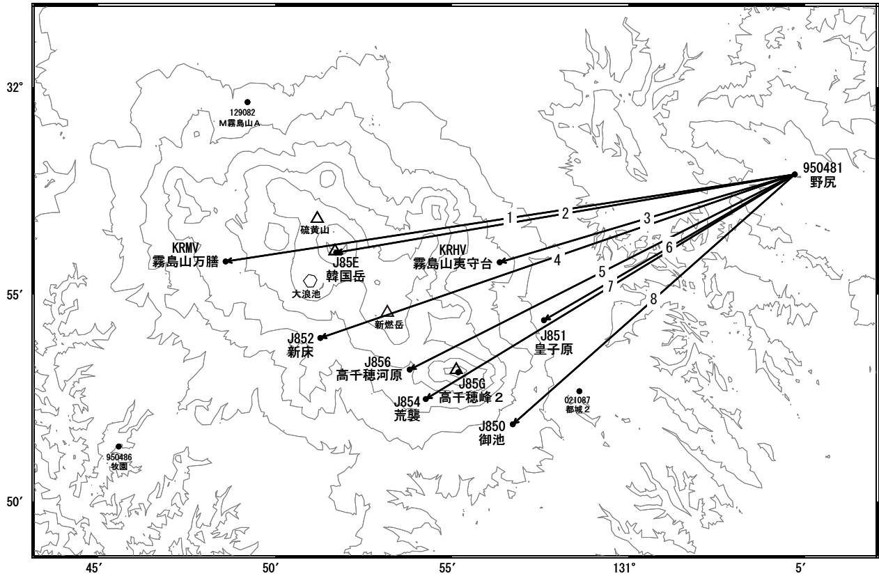
第3図 霧島山周辺のGNSS連続観測結果・統合解析基線配置図
