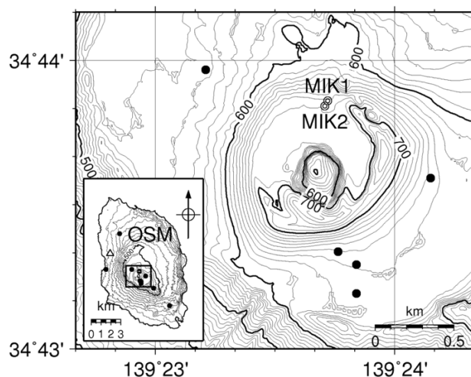
第1図 三原山火口付近と伊豆大島全域の全磁力観測点配置(○:地磁気観測所連続観測点、●:東京大学地震研究所連続観測点、△:大島特別地域気象観測所)
