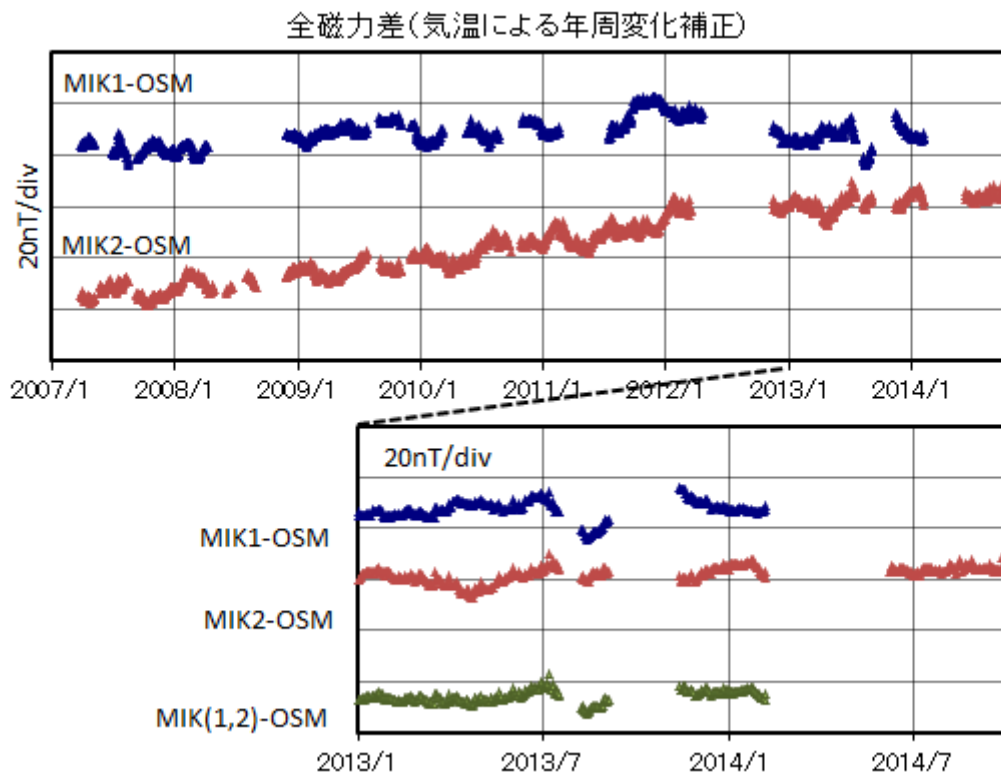
第 3 図 気温補正後の全磁力日平均値差（上図：期間 2007 年 3 月～2014 年 9 月、下図：期間 2013 年 1 月～2014 年 9 月、下図緑色：MIK1 と MIK2 の平均値）
