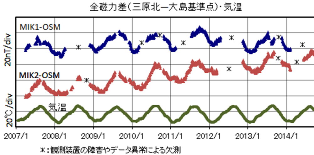
第 2 図 2007年 3 月から 2014年 9 月までの連続観測点における全磁力日平均値と参照点 OSM の日平均値との差および気温（大島特別地域気象観測所の気温データの 30 日移動平均値）
