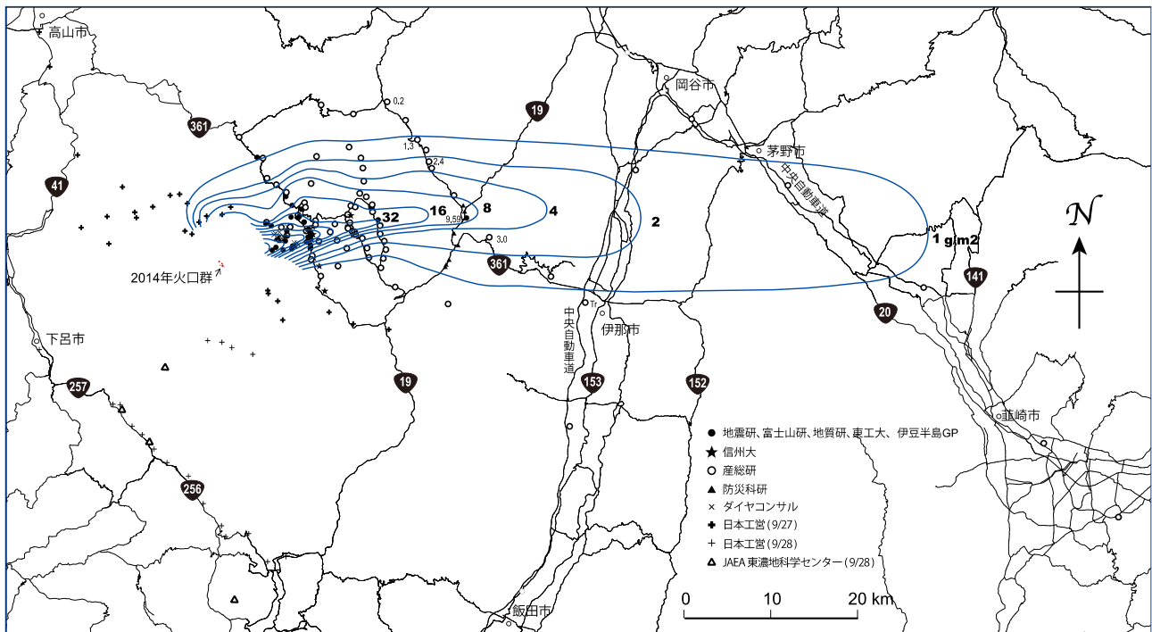
第 1 図 御嶽山 2014 年 9 月 27 日噴出物の等重量線図
