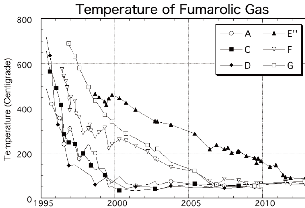
第3図 平成新山ドームの噴気ガスの温度変化。 Fig. 3. Temperature of fumarolic gas observed on the Heisei-Shinzan lava dome.
