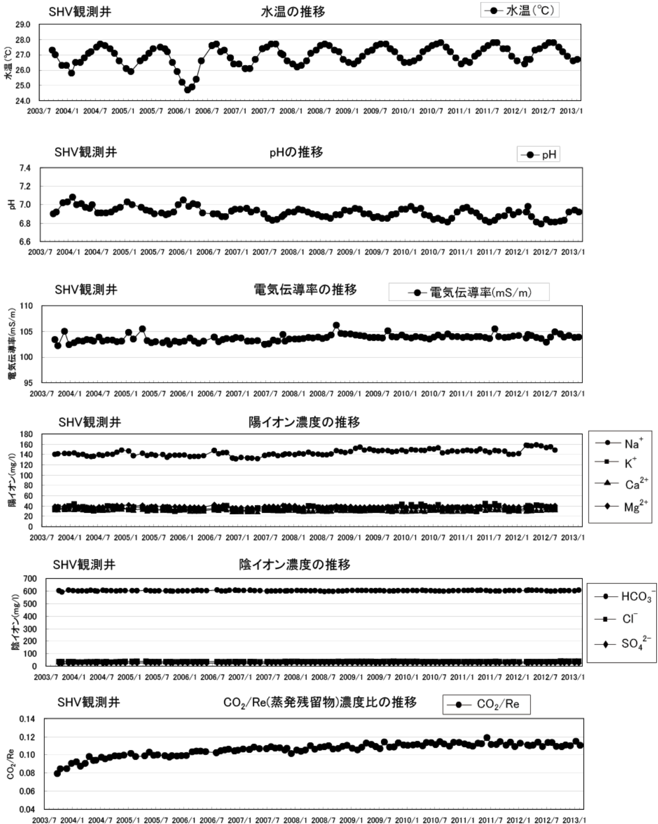
第5図 SHV観測井の水温・pH・電気伝導率・主要化学成分濃度・CO 2 /Re(蒸発残留物)濃度比の推移。
