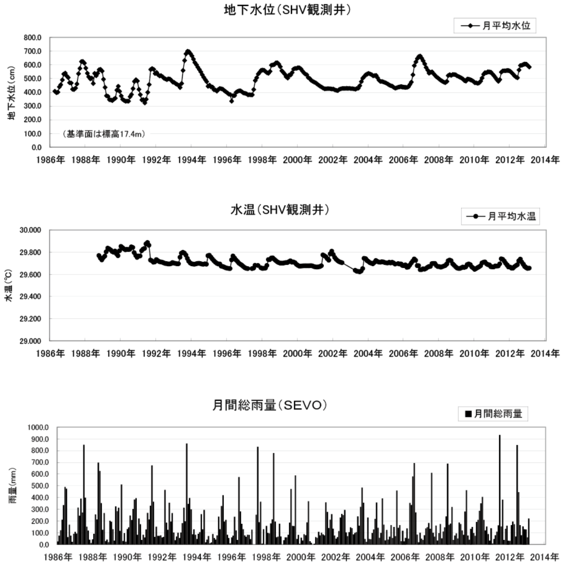
第4図 SHV 観測井における月平均水位・月平均水温・月間総雨量の観測結果。2005年5月以降の月間総雨量は気象庁アメダス島原を使用。
