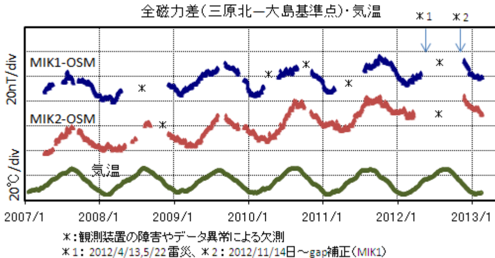
第2図 2007年3月から2013年2月までの連続観測点における全磁力日平均値と参照点OSMの日平均値との差および気温（大島特別地域気象観測所の気温データの30日移動平均値）
