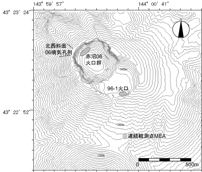
第1図 全磁力観測点配置図 (◎連続観測点MEA)
