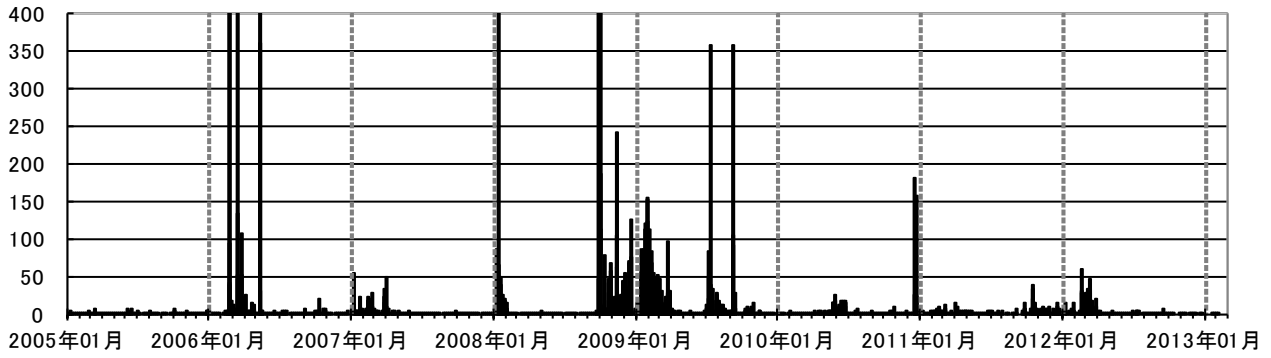
第6図 オンネトー南東観測点における地震日回数（2005年1月1日～2013年2月10日）
