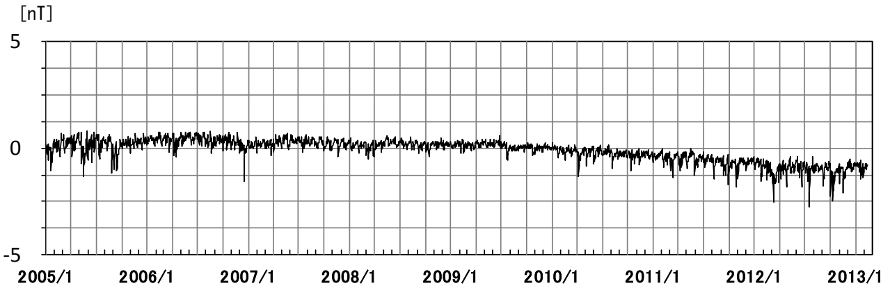
第4図 MMBの地磁気水平成分から求めた太陽活動等によるノイズ量(2005年1月1日~2013年2月10日)
