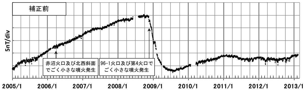
第2図 MEAにおける全磁力日平均値とMMBの全磁力日平均値との差(2005年1月1日～2013年2月10日)
