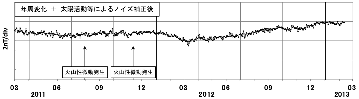
第7図 MEAとMMBの年周変化補正と太陽活動等によるノイズ補正後の全磁力日平均値差（2011年3月1日～2013年2月10日）
