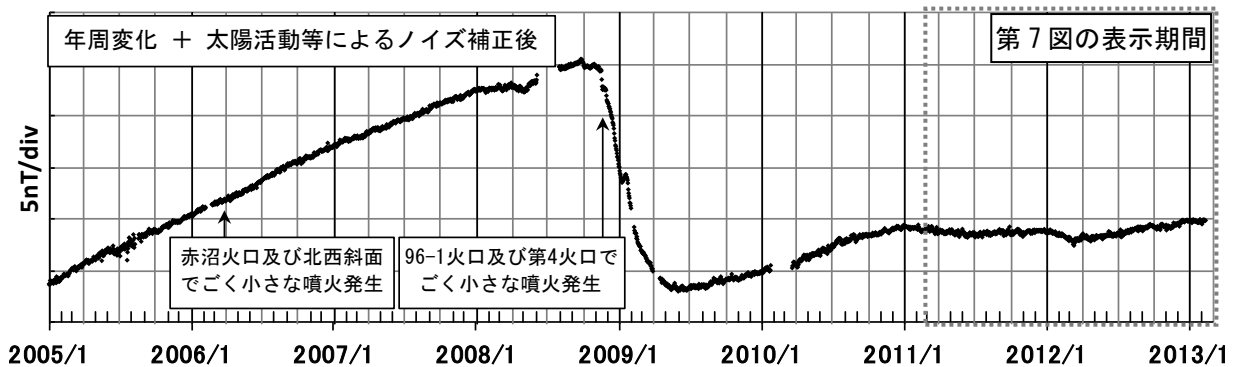
第5図 MEAとMMBの年周変化補正と太陽活動等によるノイズ補正後の全磁力日平均値差(2005年1月1日~2013年2月10日)
