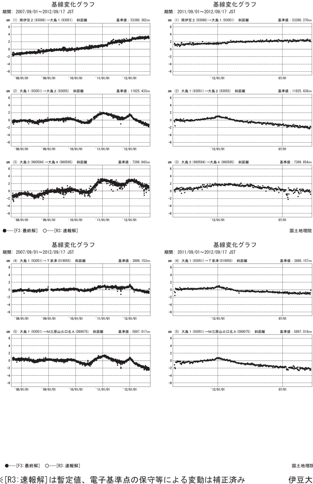
第2図 (a) 伊豆大島のGNSS連続観測結果(基線長:左列2007年9月~2012年9月、右列2011年9月~2012年9月)
