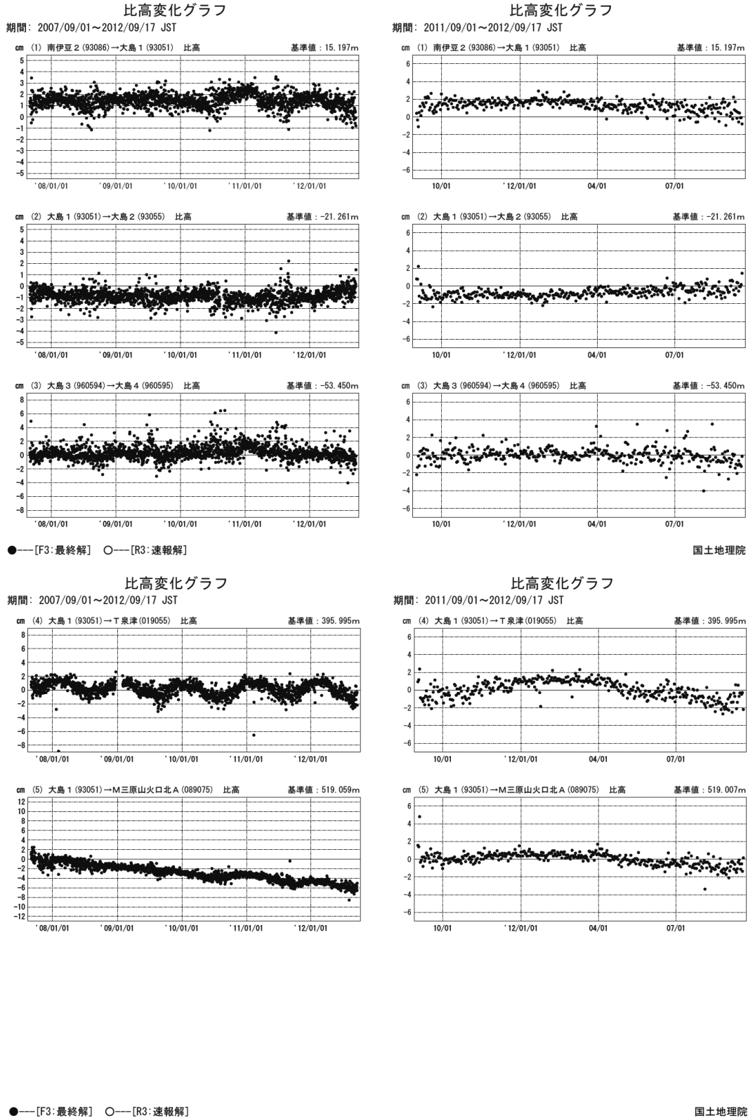
第2図 (b) 伊豆大島のGNSS連続観測結果 (比高: 左列 2007年9月~2012年9月、右列 2011年9月~2012年9月)
