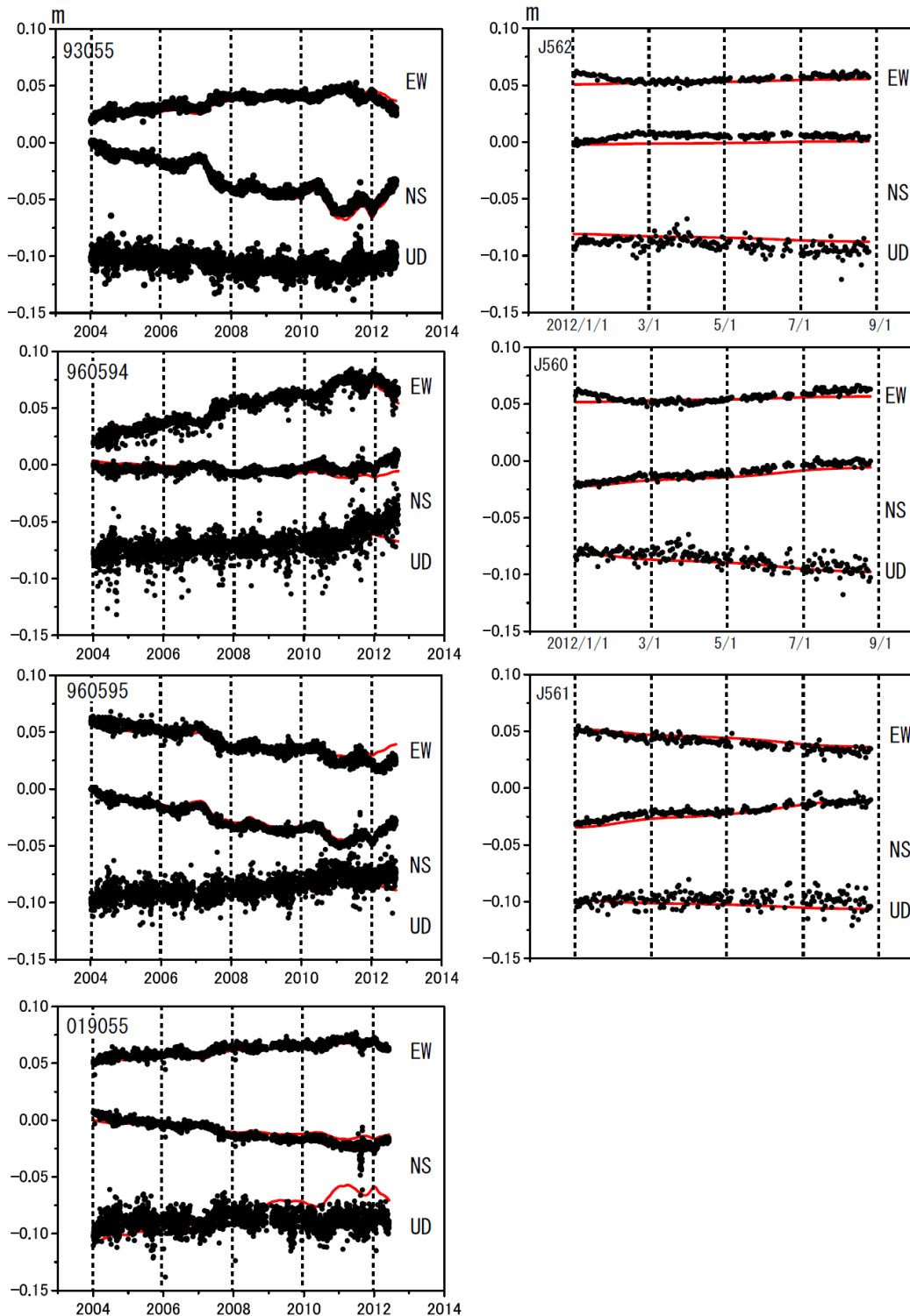
第7図 推定された茂木ソースによる地殻変動計算値(赤実線)と観測値(黒点)の比較
