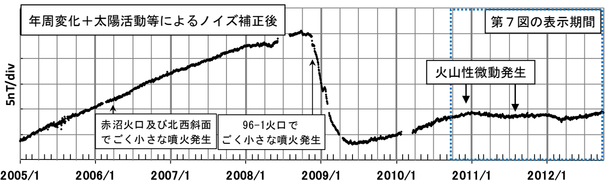
第5図 MEAとMMBの年周変化補正と太陽活動等によるノイズ補正後の全磁力日平均値差(2005年1月~2012年9月)
