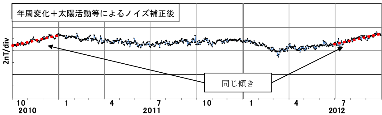
第7図 MEAとMMBの年周変化補正と太陽活動等によるノイズ補正後の全磁力日平均値差 (2010年10月～2012年9月)
