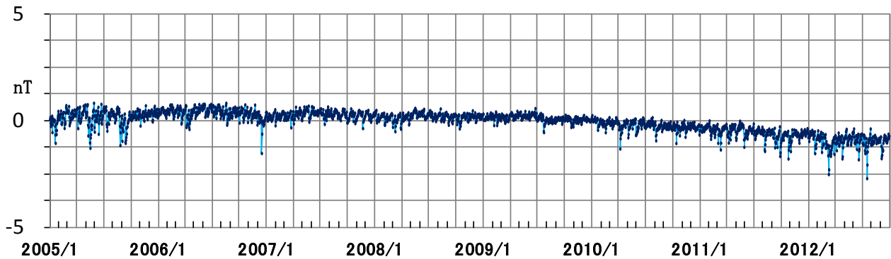
第4図 MMBの地磁気水平成分から求めた太陽活動等によるノイズ量(2005年1月~2012年9月)
