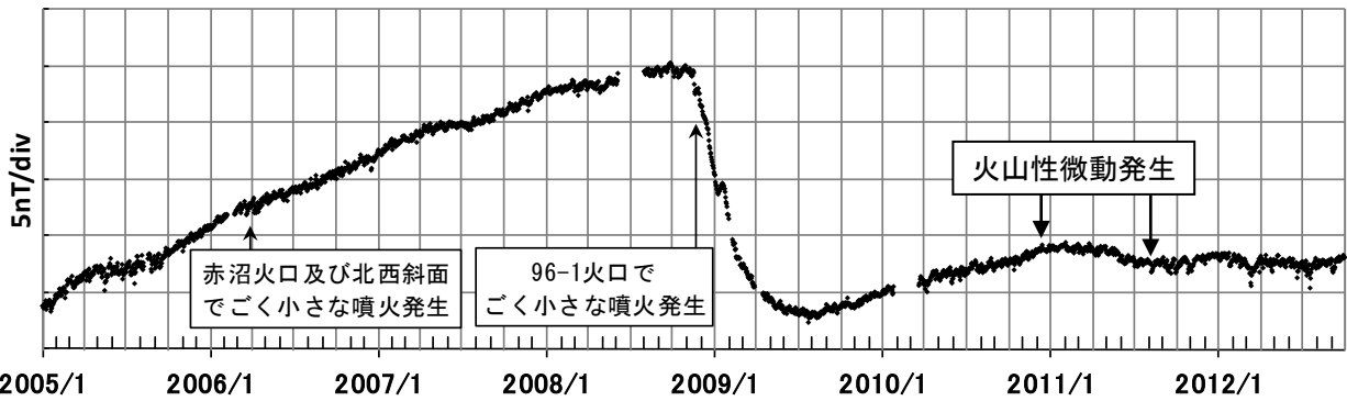
第2図 MEAにおける全磁力日平均値とMMBの全磁力日平均値との差 (2005年1月～2012年9月) Fig.2 Daily mean differences of the geomagnetic total intensity at MEA from that at MMB from January 2005 to September 2012.
