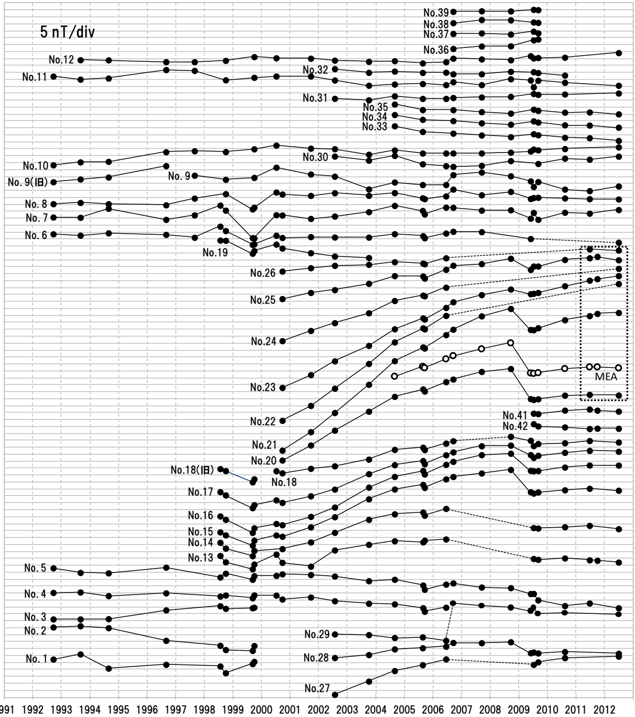
第8図 繰り返し観測点における全磁力とMMBの全磁力との差（1992年9月～2012年6月）
