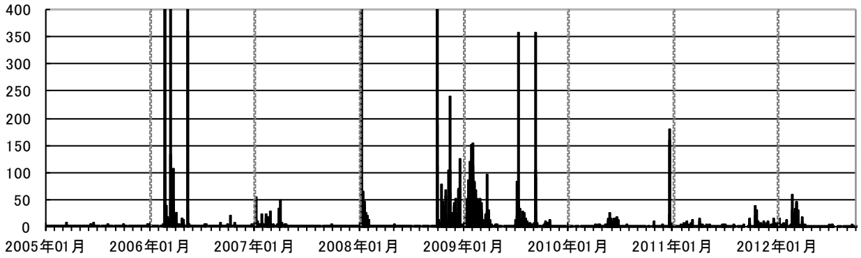
第6図 オンネトー南東観測点における地震日回数 (2005年1月～2012年9月)
