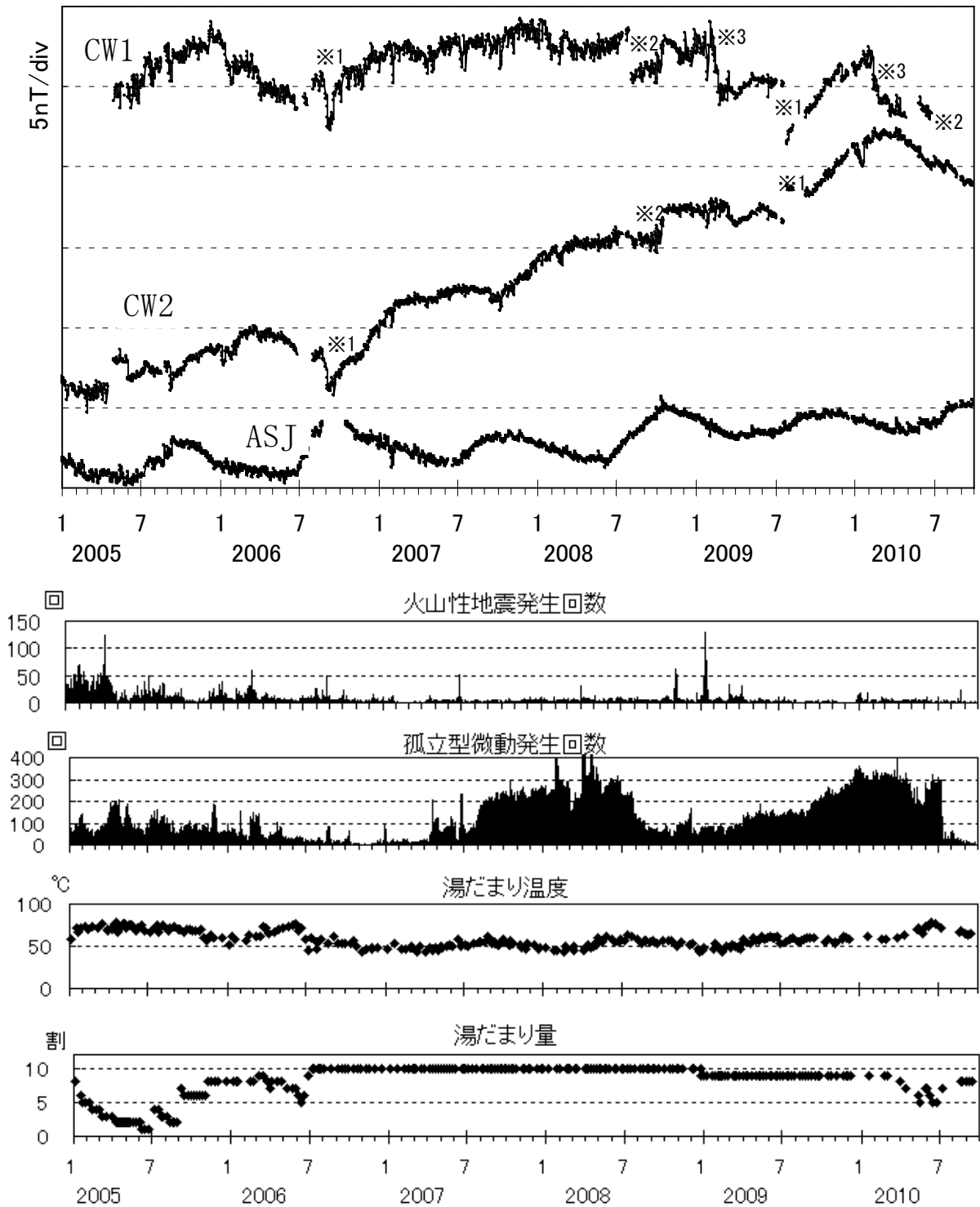
第2図 2005年1月から2010年9月までの連続観測点CW1、CW2、ASJにおける全磁力日平均値と参照点AHKの日平均値との差、火山性地震発生回数、孤立型微動発生回数、湯だまり温度、湯だまり量。 ※1の変化の原因は不明。 ※2の変化は磁力計の不具合と思われる。 ※3の変化は検出器周辺の土砂の移動が原因と思われる。
