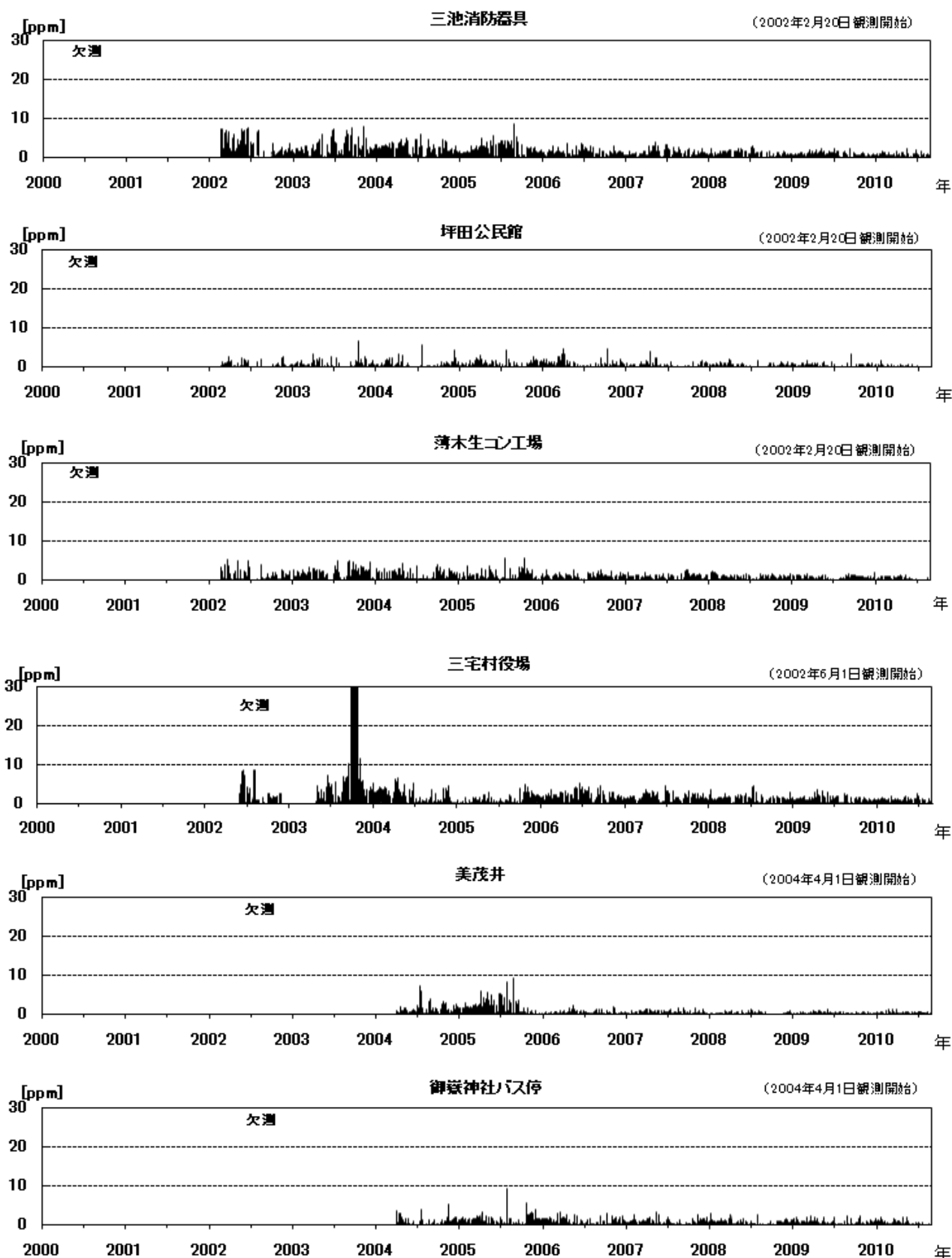
第 8 図※-② 三宅島火山ガス観測結果（一時間値）（2000 年～2010 年 8 月）
