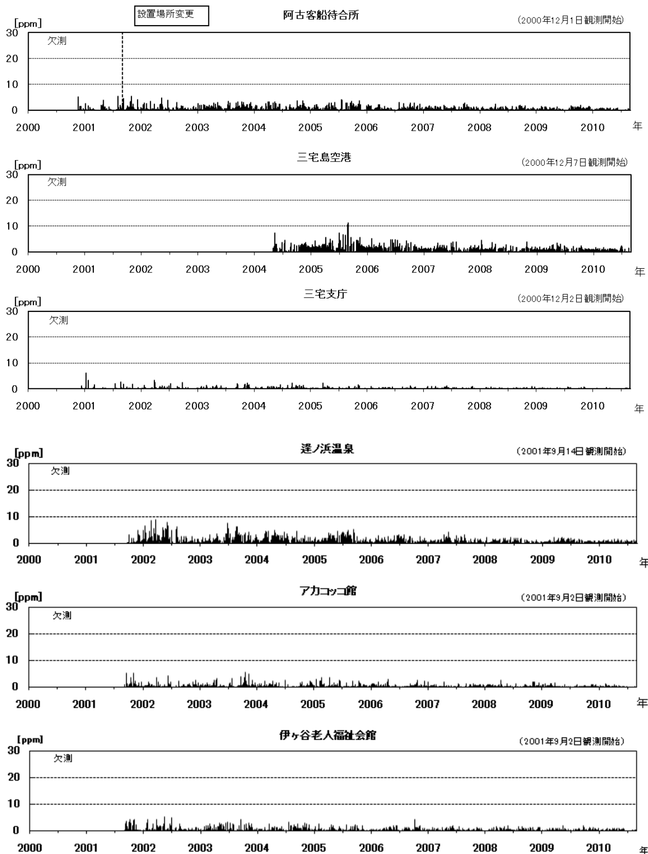
第 8 図※—① 三宅島火山ガス観測結果（一時間値）（2000 年～2010 年 8 月） グラフは三宅村から提供された火山ガスデータをもとに気象庁が作成。
