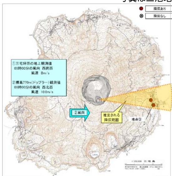
第5図 三宅島 7月21日 09時28分頃の噴火に伴う降灰の状況 写真は三宅村営バス駐車場(地点③)での状況
