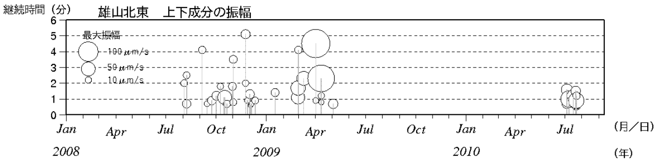
第 10 図 三宅島 火山性微動活動経過図 (2008 年 1 月 1 日~2010 年 9 月 10 日) ・ 7 月に火山性微動が計 11 回発生した。
