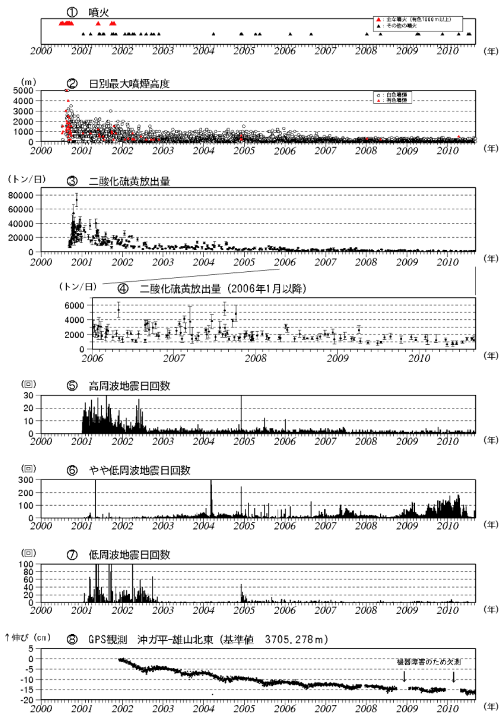
第6図※ 三宅島 火山活動経過図 (2000年1月1日～2010年9月10日)
