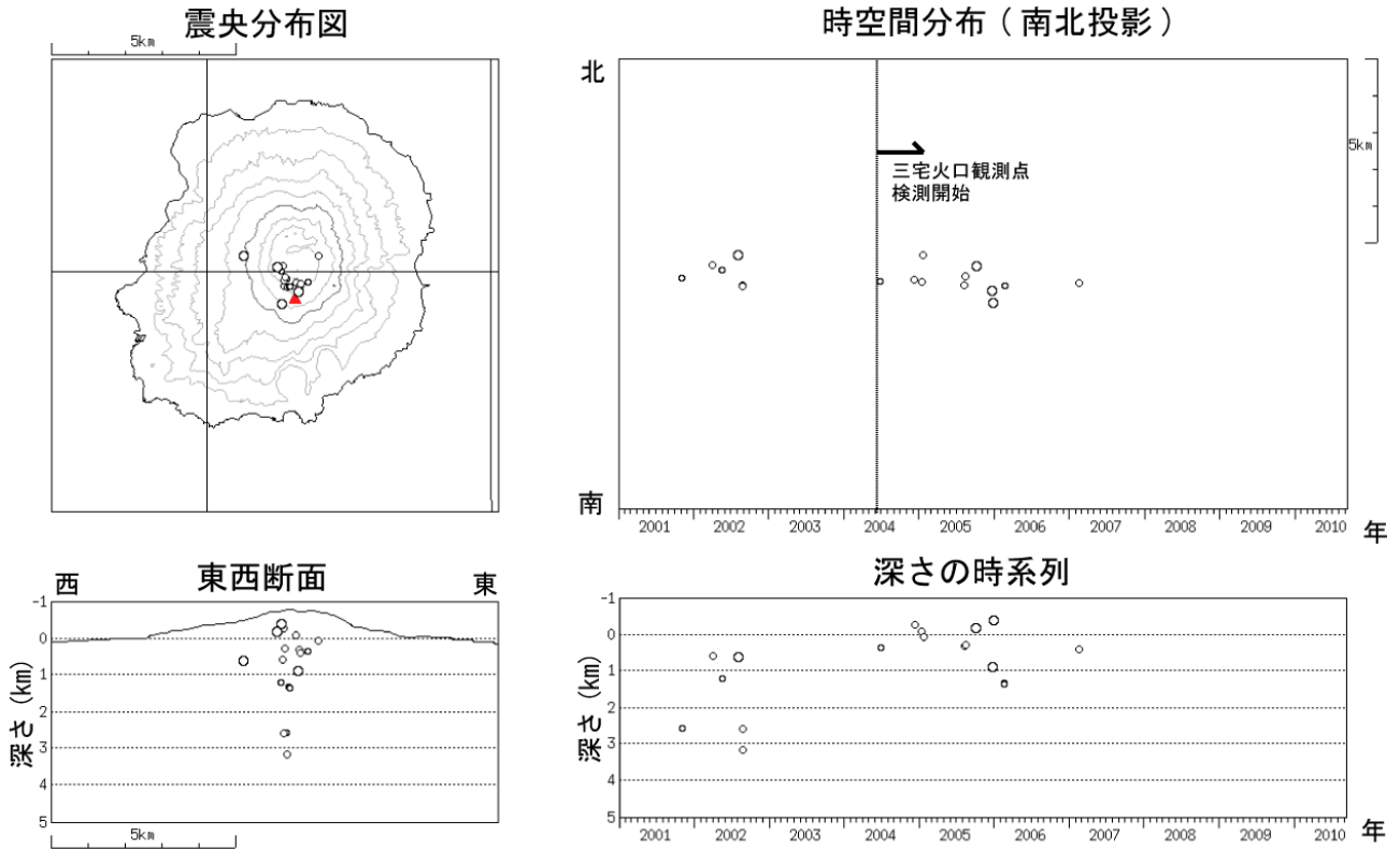
第 9 図-③ 三宅島 低周波地震の震源分布 (2001 年 1 月 1 日~2010 年 9 月 10 日) ○ : 2001 年 1 月 1 日~2010 年 5 月 31 日 ● : 2010 年 6 月 1 日~2010 年 9 月 10 日 注) 図 6-①~③では、震源計算には半無限速度構造 ( V_p=2.5\text{km/s} 、 V_p/V_s=1.73 ) を使用。 この地図の作成には、国土地理院発行の『数値地図 50mメッシュ (標高)』を使用した。 ・震源はこれまでと同様、山頂直下の浅部に分布した。
