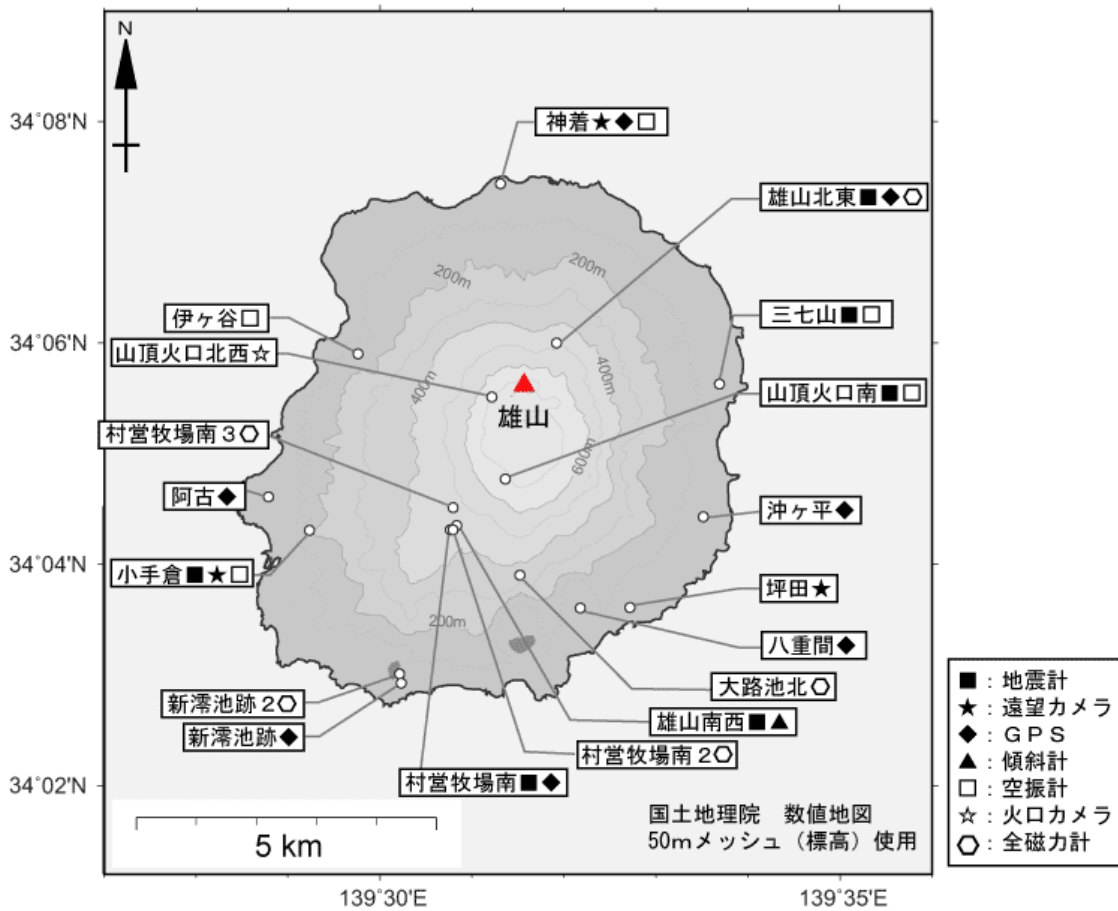
第1図 三宅島 気象庁の観測点配置図
