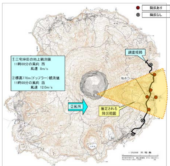
第3図 7月4日 10時19分の噴火に伴う降灰の状況 写真は三宅村役場(地点①)での状況
