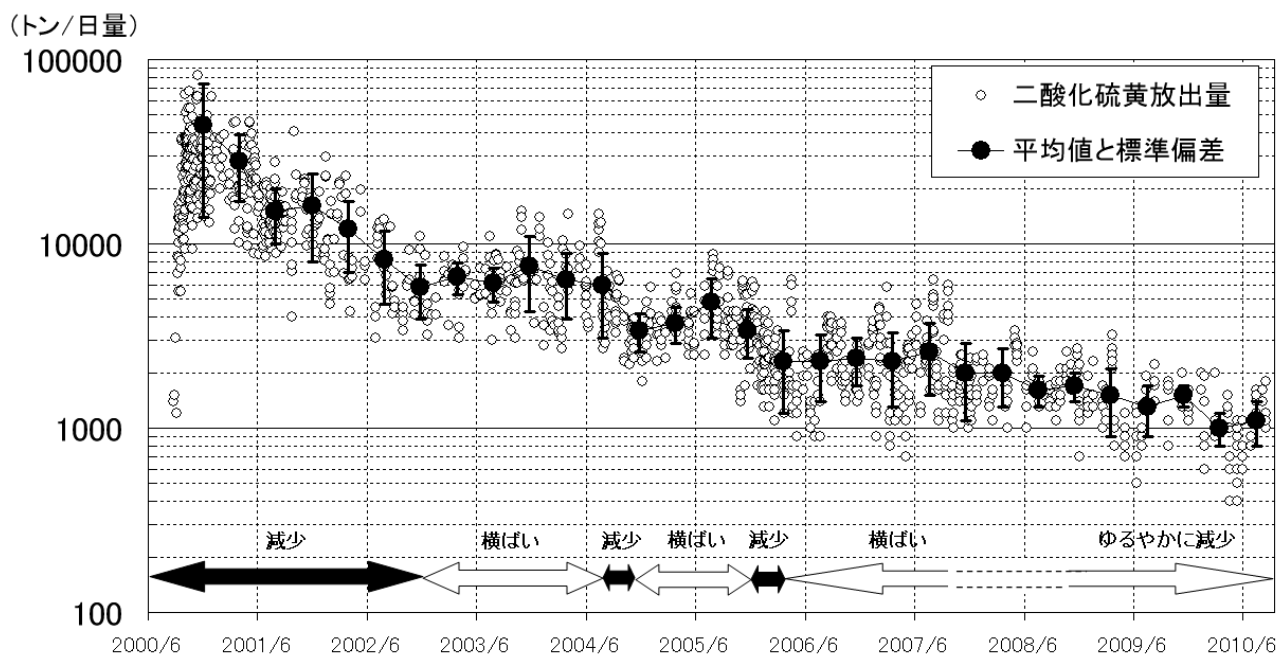
第7図※ 三宅島 二酸化硫黄放出量と平均値の推移 (図3-③を対数スケールで表示)
