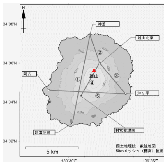
第11図 三宅島 GPS連続観測による基線長変化 (2000年10月～2010年9月10日)
