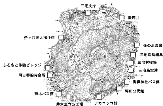
第 8 図※-③ 三宅島火山ガス観測結果（一時間値）と三宅島測候所の風向風速（気象庁） (2000 年～2010 年 8 月) および三宅村火山ガス観測点配置図 グラフは三宅村から提供された火山ガスデータをもとに気象庁が作成 この地図の作成には、国土地理院発行の『2万5千分の1地形図（三宅島）』を使用した。
