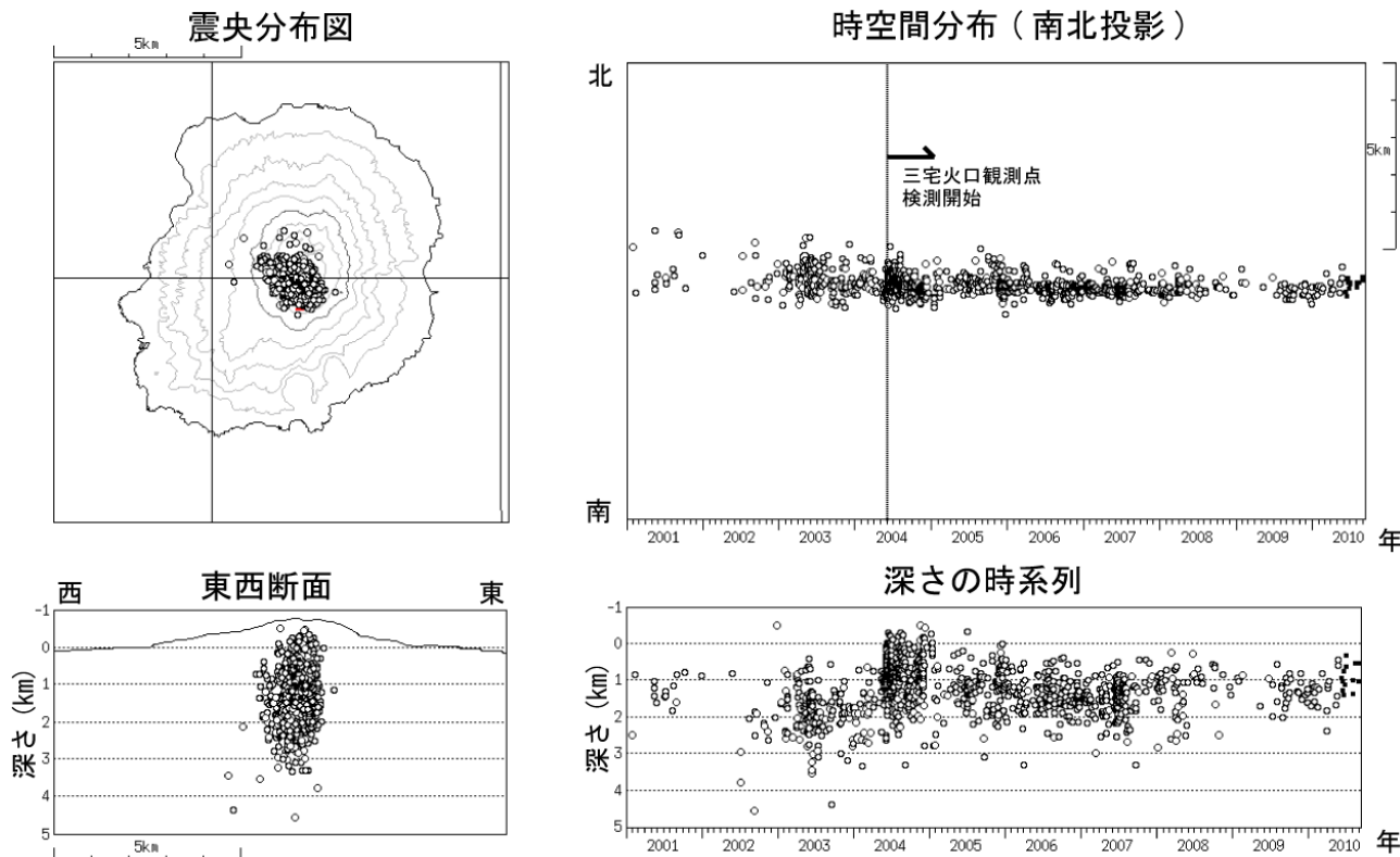
第 9 図-② 三宅島 やや低周波地震の震源分布 (2001 年 1 月 1 日~2010 年 9 月 10 日) ○ : 2001 年 1 月 1 日~2010 年 5 月 31 日 ● : 2010 年 6 月 1 日~2010 年 9 月 10 日 この地図の作成には、国土地理院発行の『数値地図 50mメッシュ (標高)』を使用した。
