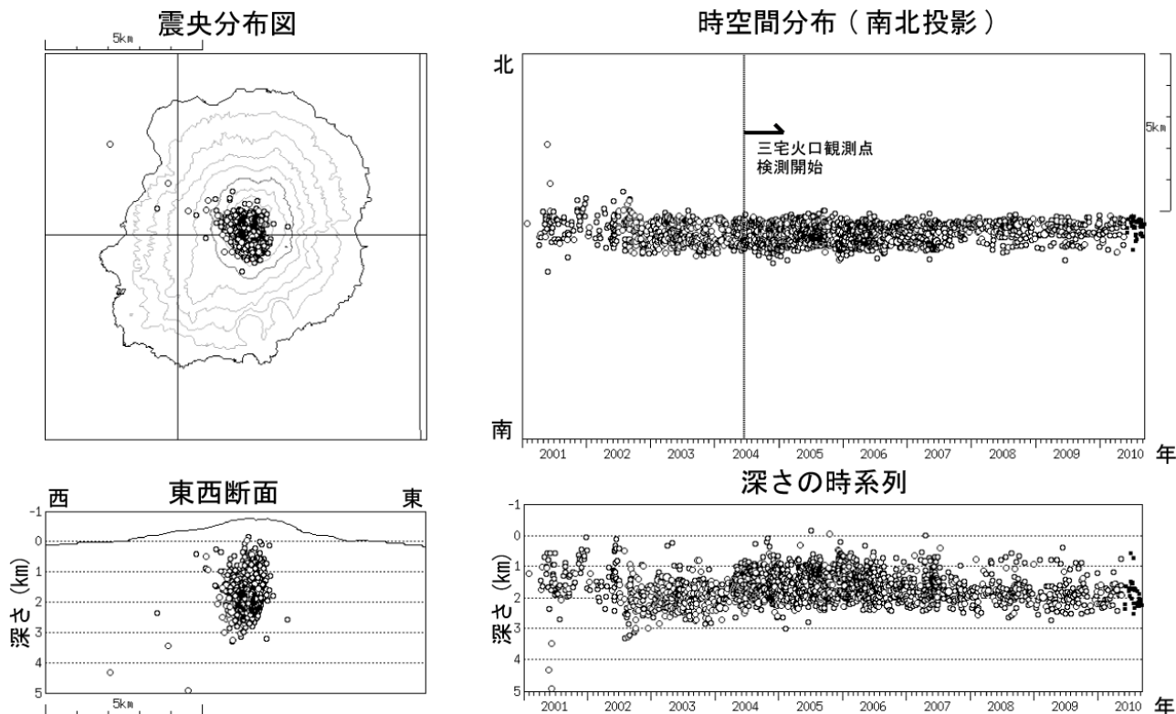
第 9 図※-① 三宅島 高周波地震の震源分布 (2001 年 1 月 1 日~2010 年 9 月 10 日) ○ : 2001 年 1 月 1 日~2010 年 5 月 31 日 ● : 2010 年 6 月 1 日~2010 年 9 月 10 日 この地図の作成には、国土地理院発行の『数値地図 50mメッシュ (標高)』を使用した。
