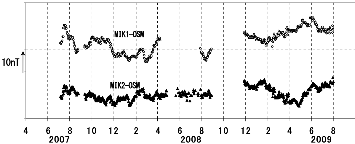
第3図 温度補正後の全磁力日平均値差 全磁力日平均値差MIK1-OSM(O)、MIK2-OSM(▲)に地中温度を用いて補正を行った値
