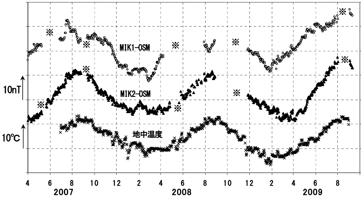
第2図 2007年4月から2009年9月までの連続観測点MIK1、MIK2における全磁力日平均値と参照点OSMの日平均値との差および観測点近傍の地中温度（※は観測装置の障害による欠測期間）
