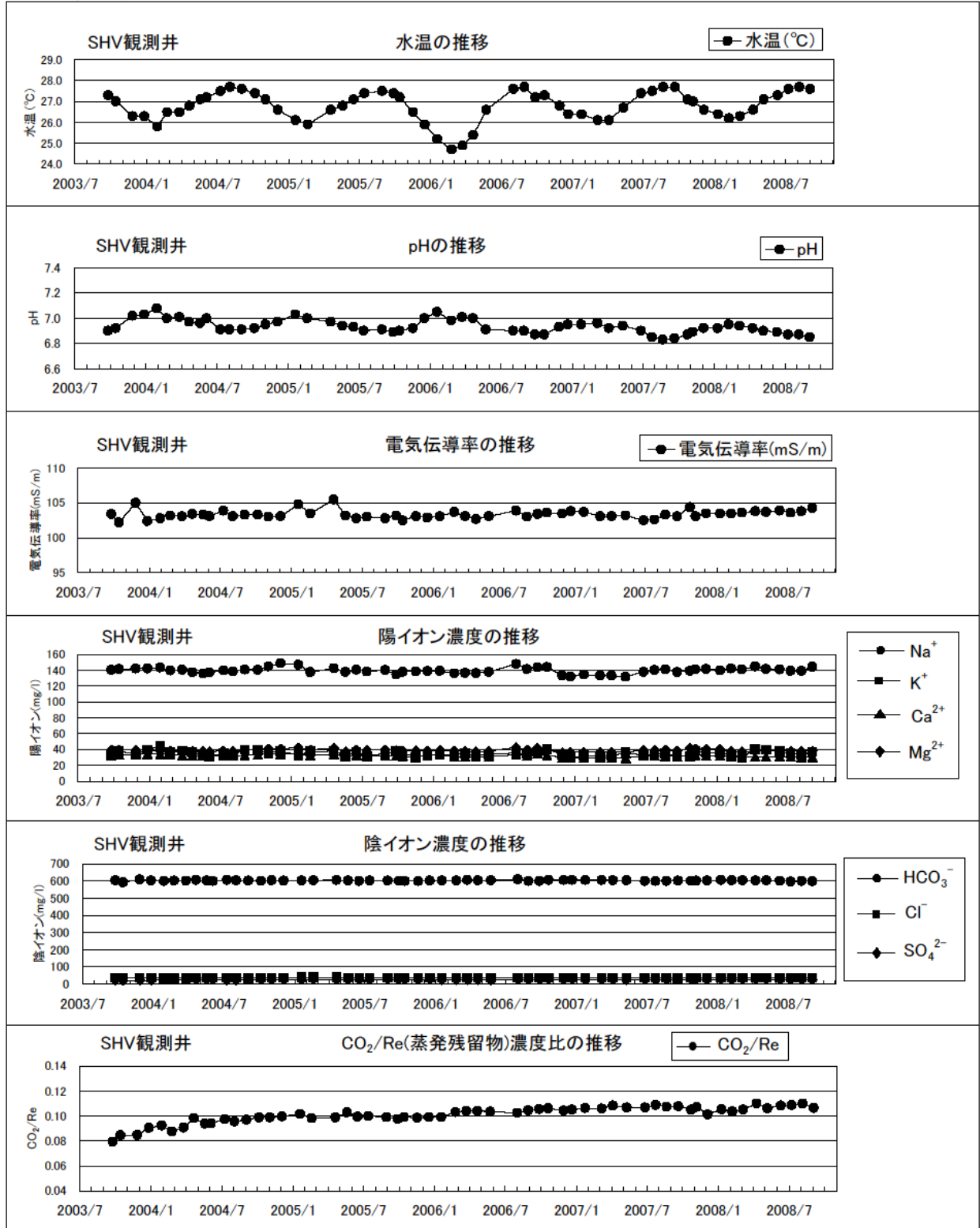
第 1 図 SHV 観測井の水温・pH・電気伝導率・主要化学成分濃度・CO 2 /Re(蒸発残留物)濃度比の推移
