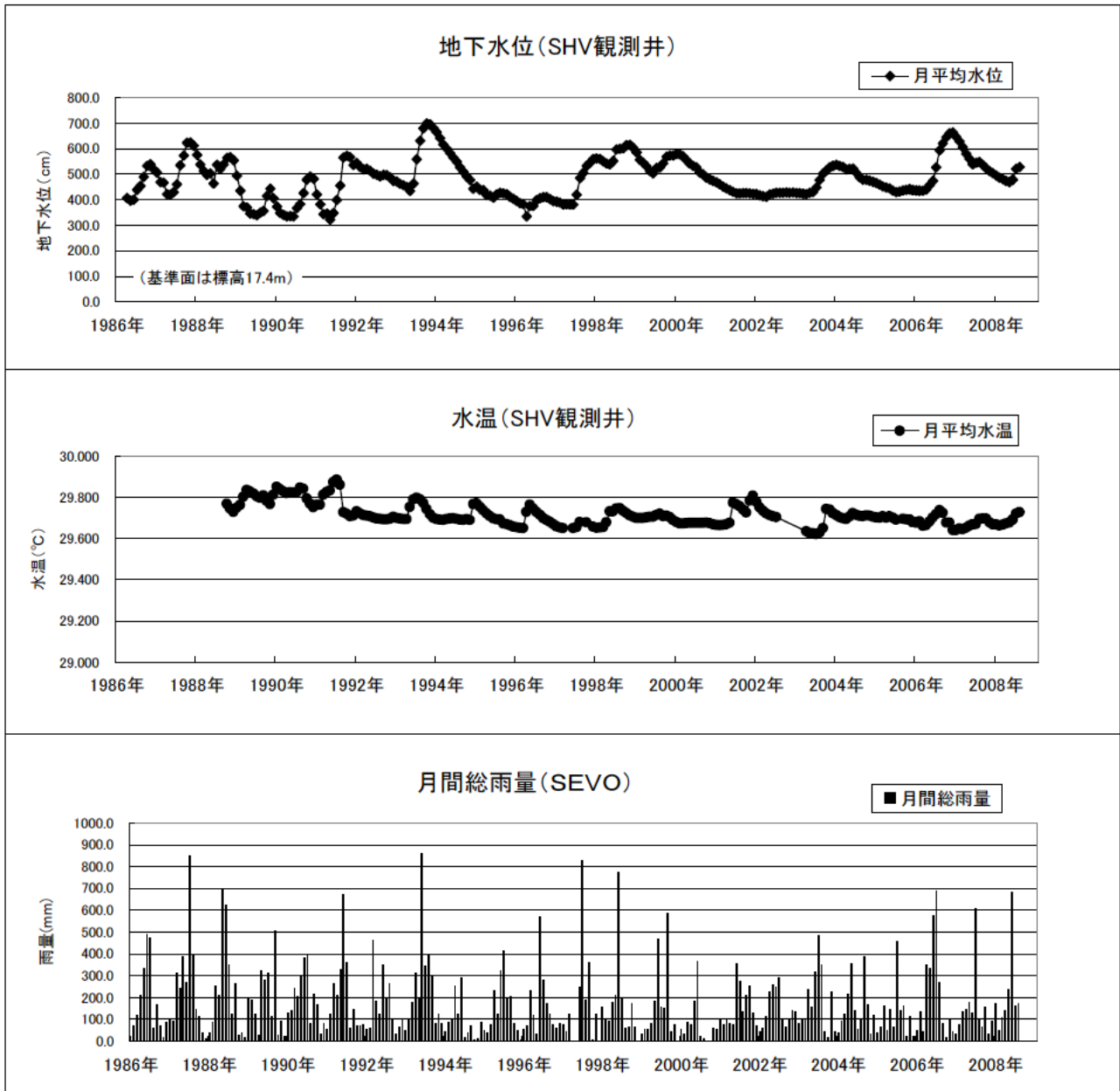
第2図 SHV 観測井における月平均水位・月平均水温・月間総雨量の観測結果. 2005年5月以降の月間総雨量は気象庁アメダス島原を使用.
