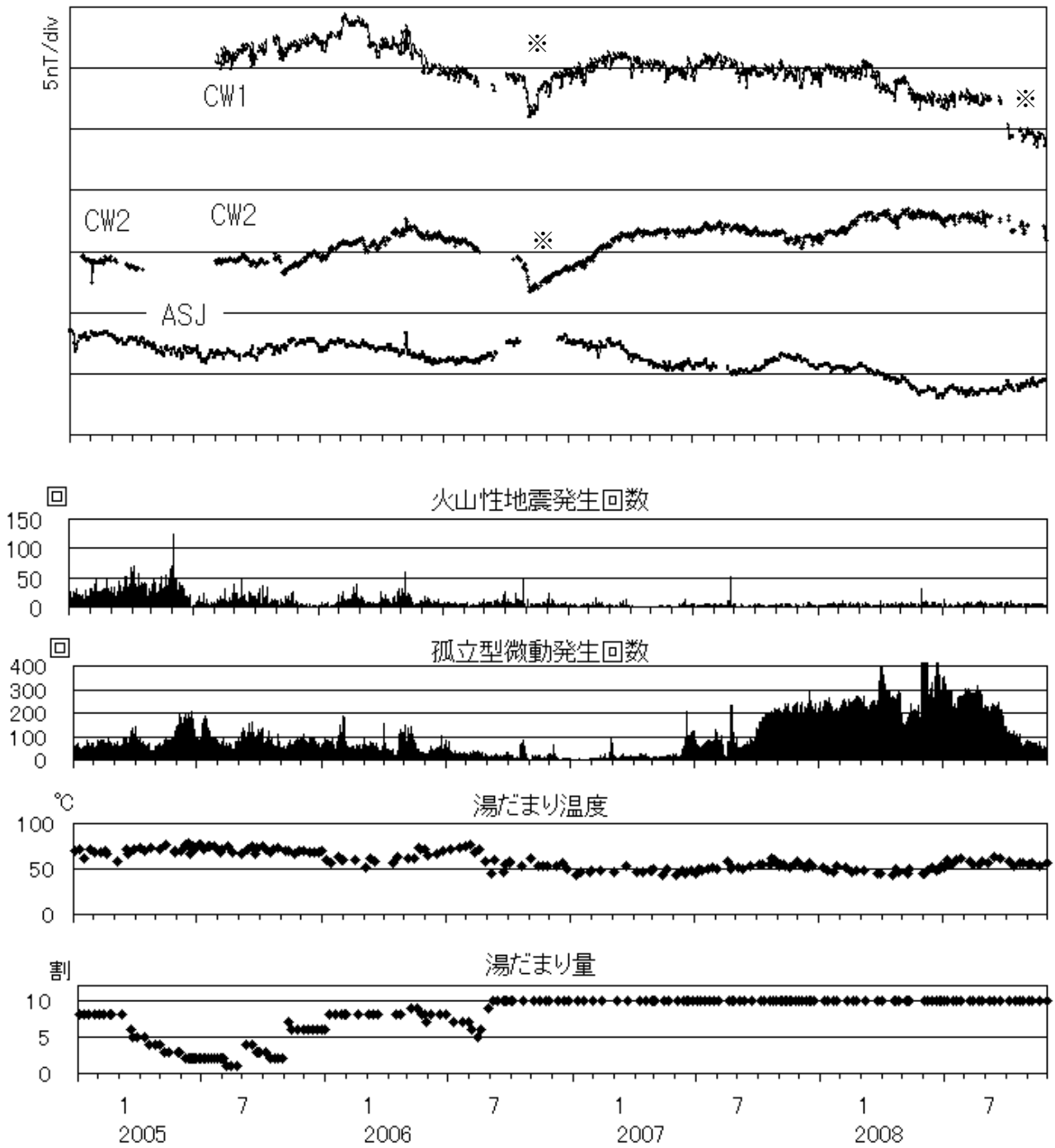
第3図 連続観測点CW1、CW2、ASJの全磁力変化からAHKの全磁力及び地磁気観測所鹿屋出張所の地磁気3成分を参照して広域の変動を除去した残差、火山性地震発生回数、孤立型微動発生回数、湯だまり温度。※印の変化の原因は不明。
