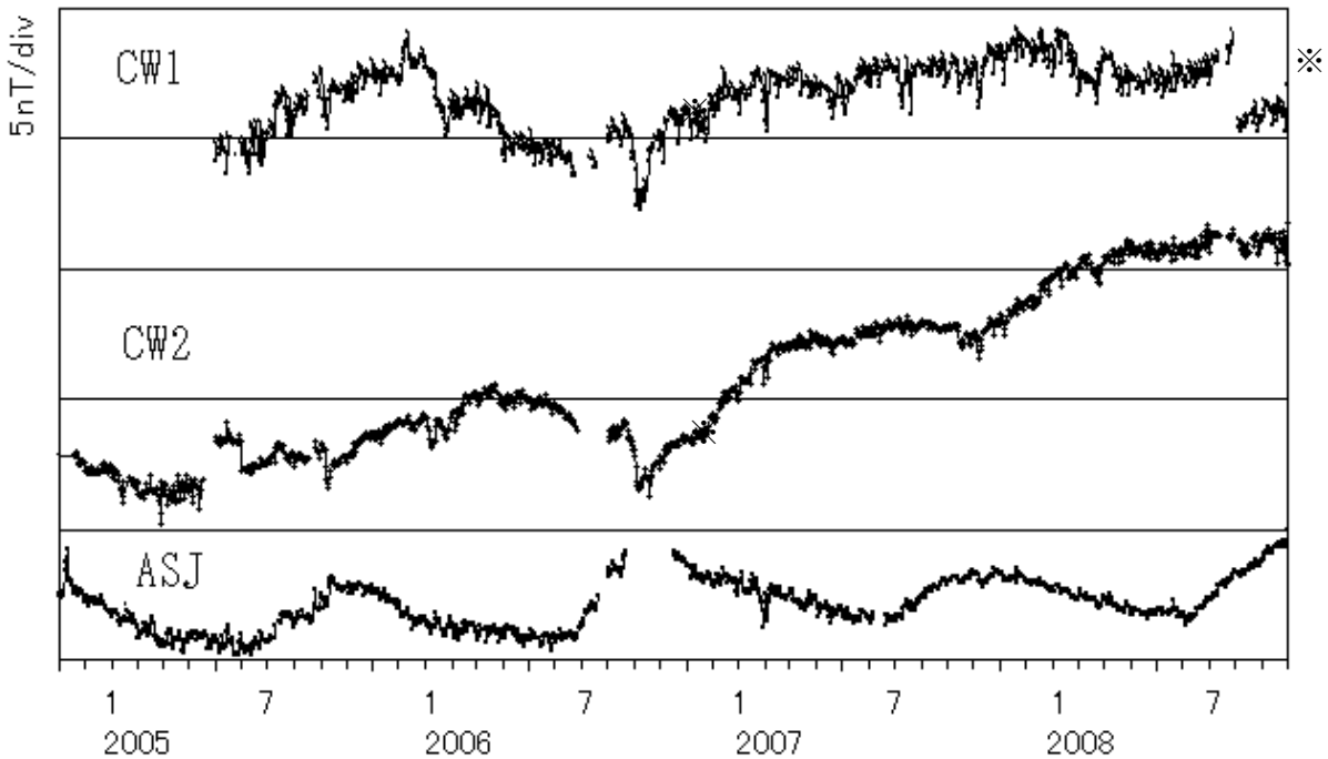
第2図 2004年11月から2008年9月までの連続観測点CW1、CW2、ASJにおける全磁力日平均値と参照点AHKの日平均値との差。*印の変化の原因は不明。
