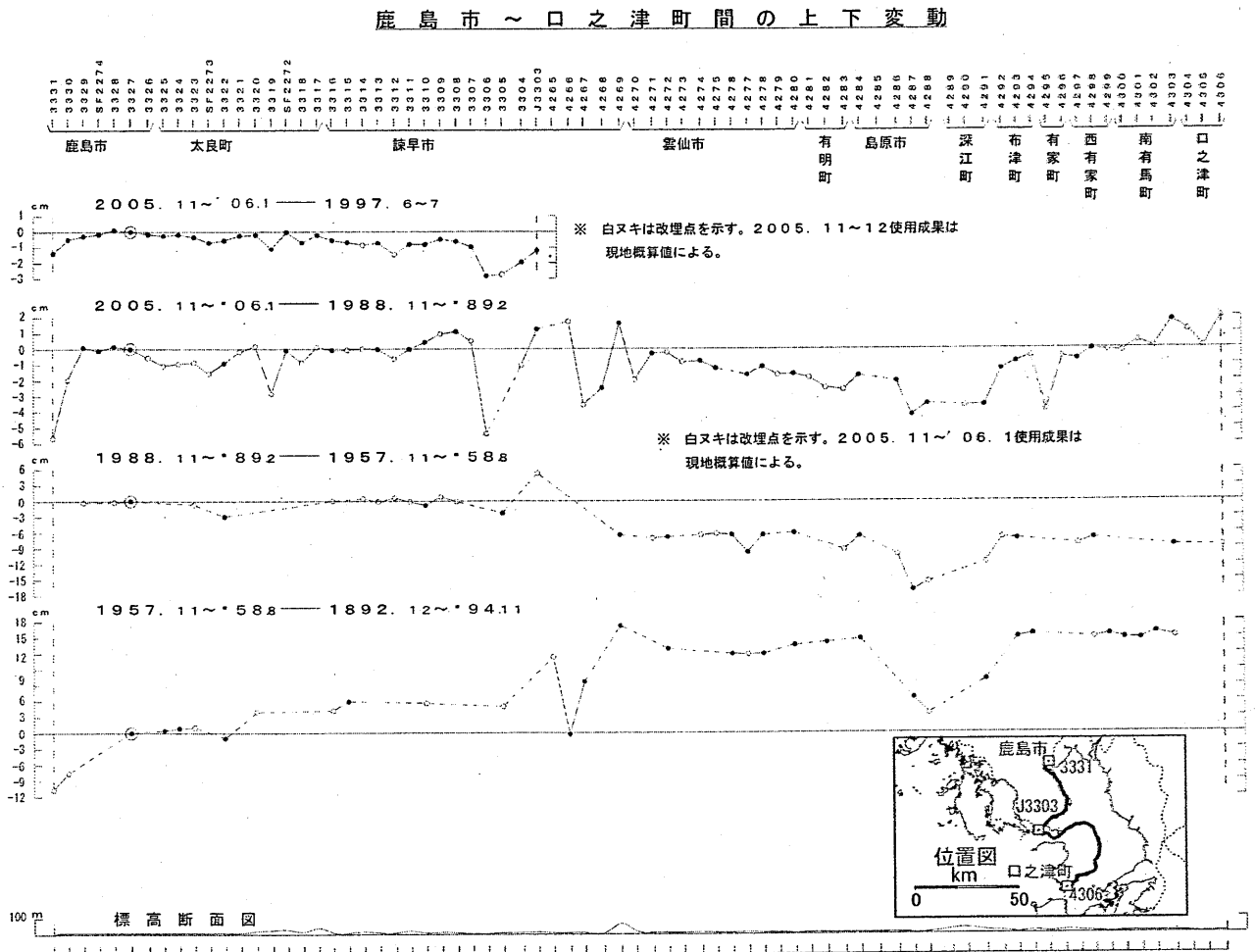
第1図 雲仙岳周辺の上下地殻変動
