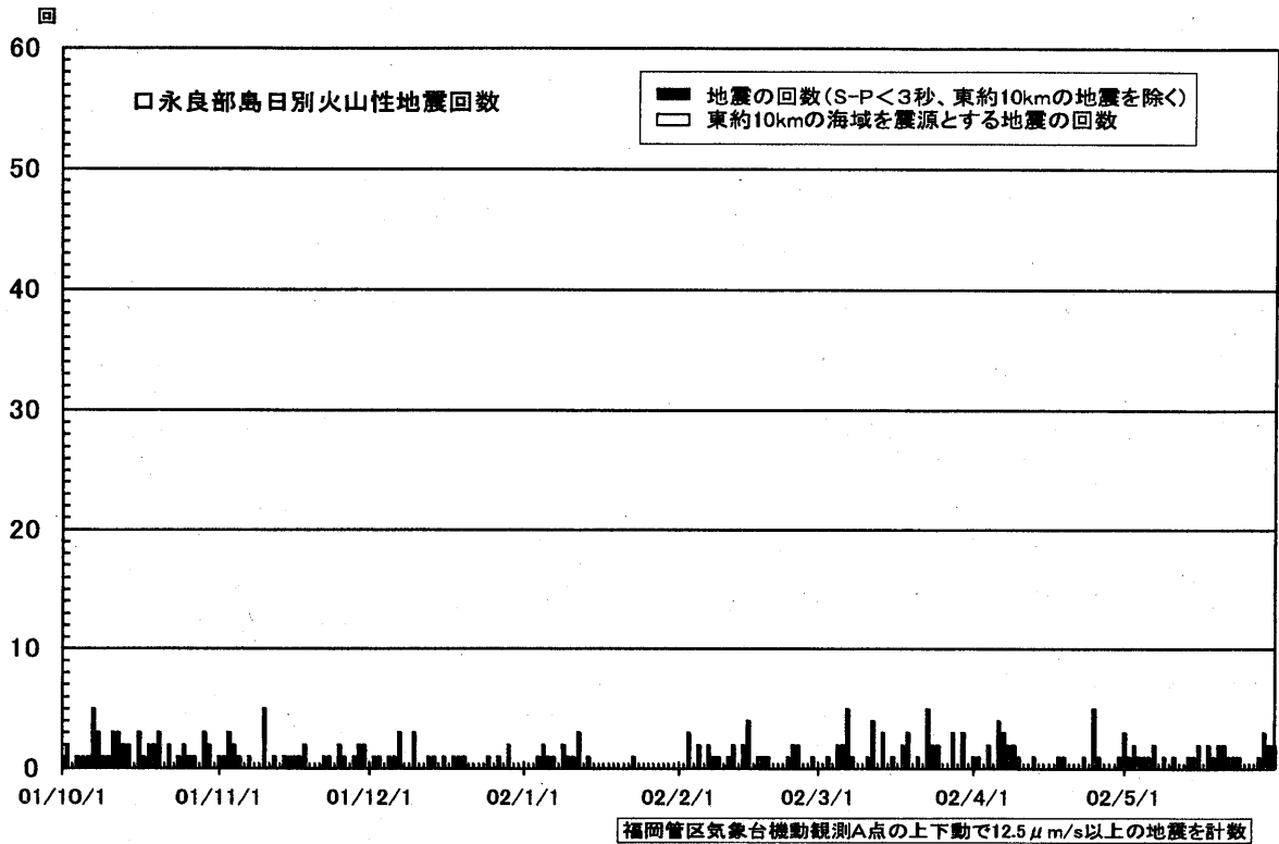
第1図 口永良部島の日別地震回数(2001年10月1日~2002年5月31日) Fig.1 Daily frequency of volcanic earthquakes at Kuchinoerabujima volcano (Oct. 1 2001 - May 31 2002).
