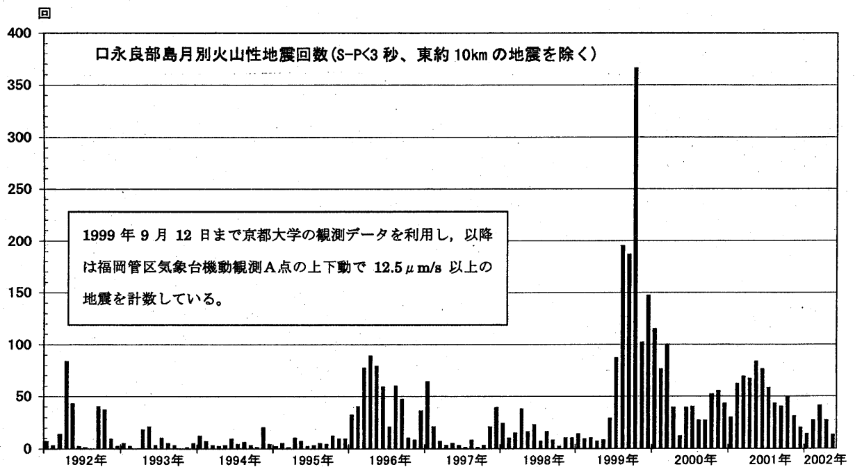
第2図 口永良部島の月別地震回数(1992年1月~2002年5月) Fig.2 Monthly frequency of volcanic earthquakes at Kuchinoerabujima volcano (Jan. 1992 - May 2002).
