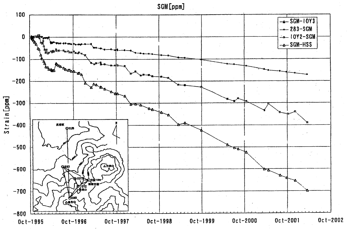
第1図 光波測量による斜距離変化(測線283-HSS、SGM-HSS、283-SGMおよびIOY-HSS) Fig.1 Changes of Distances at Io-yama Area (baseline 283-HSS, SGM-HSS, 283-SGM and IOY-HSS).
