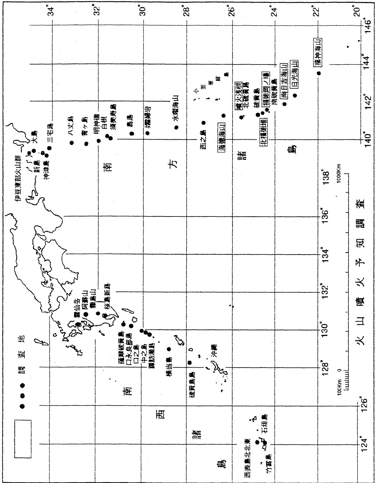
第1図 火山噴火予知調査地位位置図 Fig. 1 Index Map of submarine volcanoes and volcanic island.
