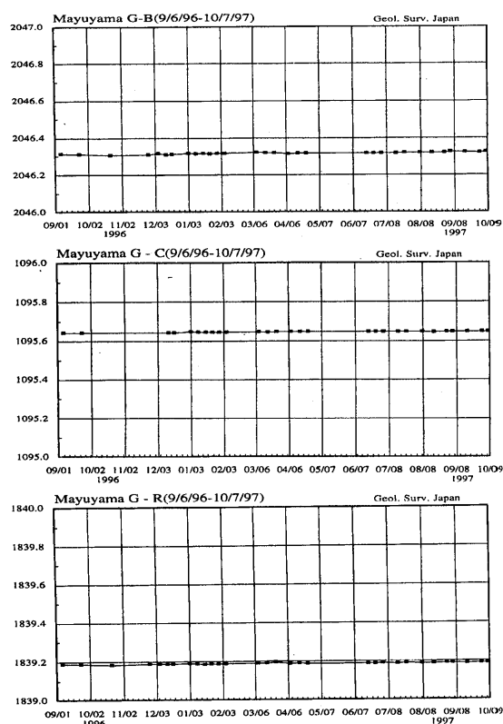
第2図 G-B、G-C及びG-R測線の斜距離変化 Fig.2 Changes in slope distances of Mayu-yama network, G-B, G-C and G-R.
