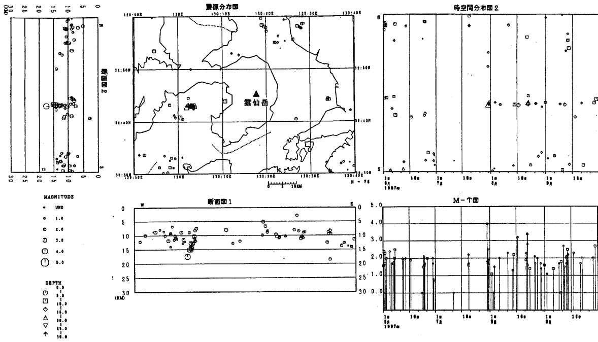
第2図 島原半島周辺の地震活動 (1997年6月1日~9月30日) Fig. 2 Seismicity around Shimabara Peninsula (1 June~30 September 1997)
