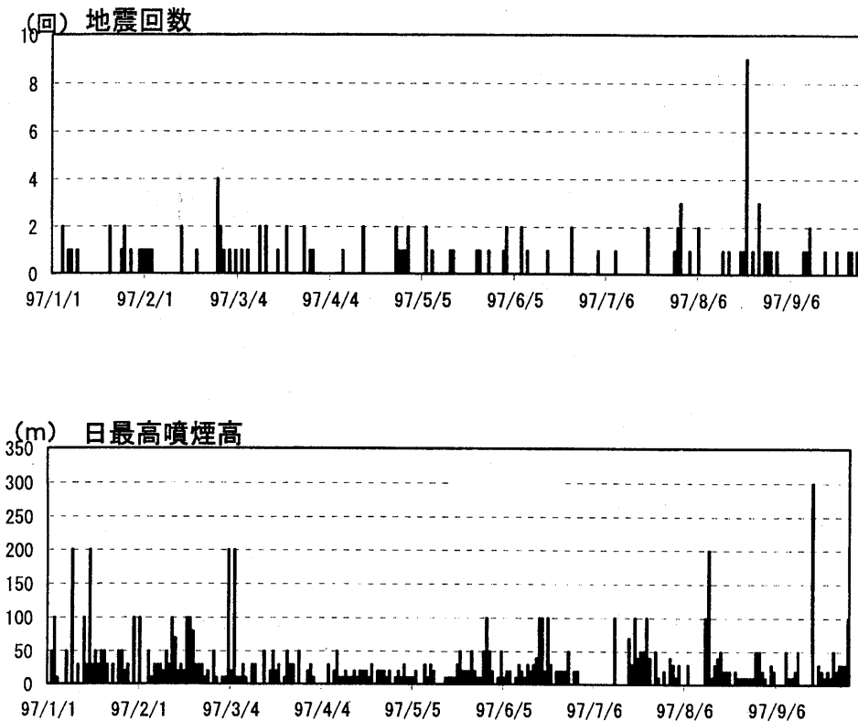
第1図 雲仙岳日別地震回数（気象庁A点地震計）（1997年1月1日～9月30日）
