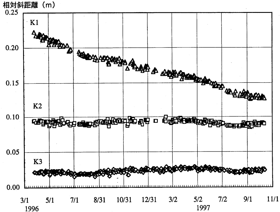
第2図 長者原-K1-3間の斜距離変化。自動連続光波測距による。日没前約2時間のデータを選択し、その平均をそれぞれ3244.70, 2782.95, 2529.45mシフトさせて表示した。 Fig.2 Change in slope distances between Chojabaru and K1 to K3 using automatic EDM system. Selected data in the stable atmospheric condition in the evening are plotted. Add 3244.70, 2782.95, and 2529.45m for each line.
