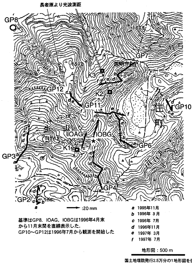
第1図 九重火山山体変動観測網。K1, K2, K3は光波測距用反射鏡, GP2-12, IOAG, IOBGはGPS観測点。矢印は1995年11月から1997年7月までのGPS観測による水平変動ベクトル。 Fig.1 Ground deformation measurement network on Kuju volcano. K1 to K3: targets for EDM, IOAG and IOBG: automatic GPS station, arrow: horizontal movement vector by GPS measurement, between November 1995 and July 1997.
