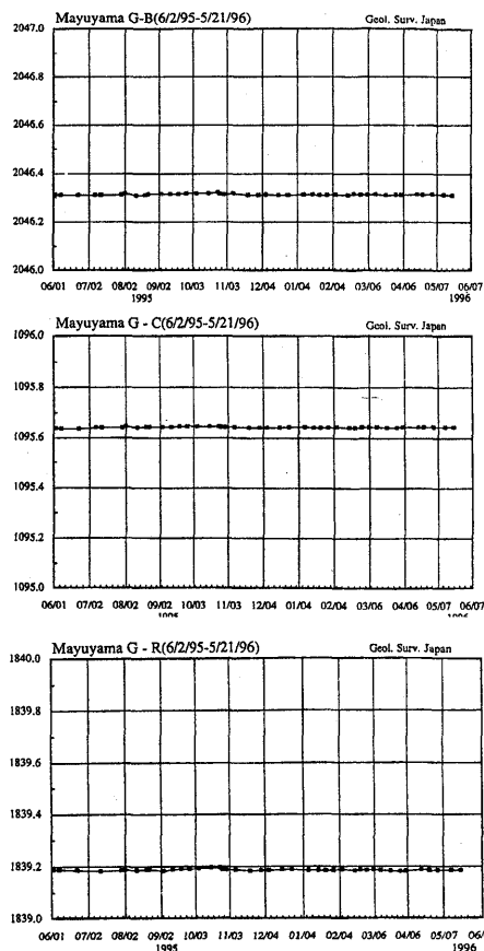
第2図 G-B、G-C及びG-R測線の斜距離変化 Fig. 2 Change in slope distance of Mayu-yama network, G-B, G-
