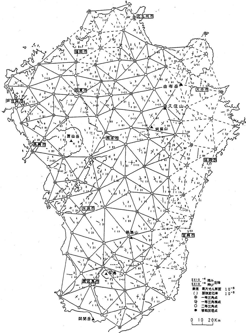
第1図 九州地方の水平歪 (1989~1991-1981~1982) Fig. 1 Horizontal crustal strain in the kyusyu district.
