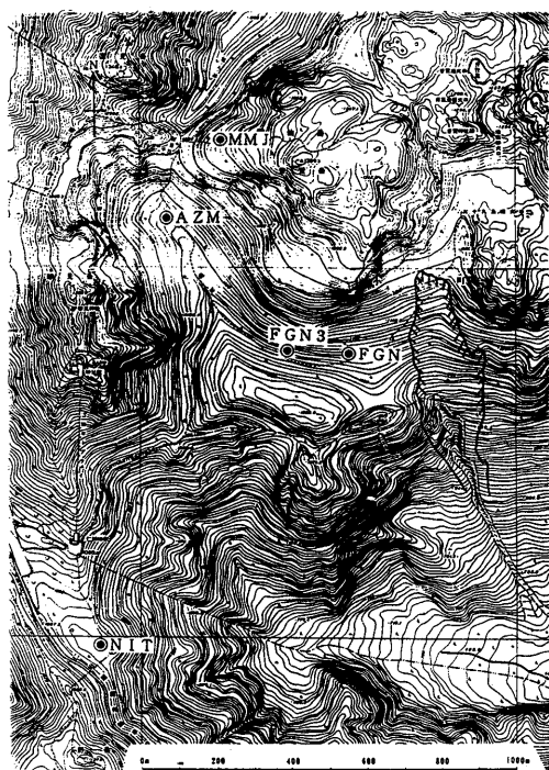
第1図 雲仙岳における全磁力連続観測開界分布及び崖崩れが発生し大規模な沢になった領域(実線で囲った部分)。普賢岳南(FGN), 普賢岳南3(FGN3), 薊谷(AZM), 紅葉谷(MMJ), 仁田峠(NIT)観測点。 Fig.1 The distribution of the continuous Observation points of the geomagnetic total force at Unzen Volcano and the area of the landslide (enclosed by a solid line).
