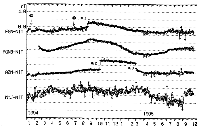
第2図 仁田峠(NIT)を基準とした各全磁力観測点における相互差(全磁力夜間値00~02時, 地磁気観測所鹿屋出張所の3成分(H, D, Z)を用いて外部磁場擾乱の影響を補正したもの)の時間的変化。
