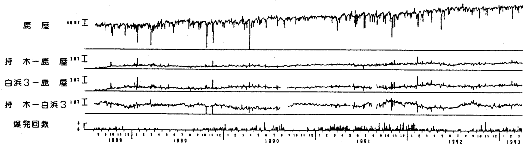
第 2 図 鹿屋の地磁気全磁力夜間値，および地磁気全磁力夜間値の相互差（持木-鹿屋，白浜3-鹿屋，持木-白浜3）の日平均値変化。下段は日別爆発回数。 （1988年8月～1993年3月）
