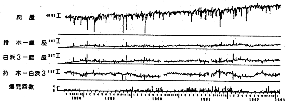
第3図 地磁気全磁力夜間値の相互差(持木-鹿屋, 白浜3-鹿屋, 持木-白浜3)の日平均値変化(1988年8月~1993年1月)
