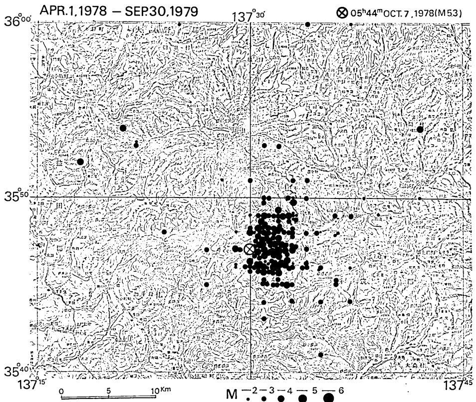
第2図 長野県王滝村付近の群発地震の震央分布図
