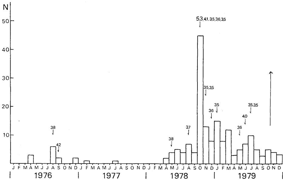
第1図 長野県王滝村付近の日別地震回数 数字は地震のマグニチュードM(3.5以上)
