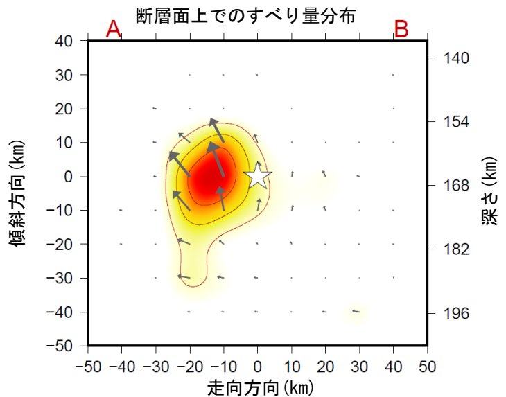
星印は破壊開始点、矢印は下盤側に対する上盤側の動きを表す。
