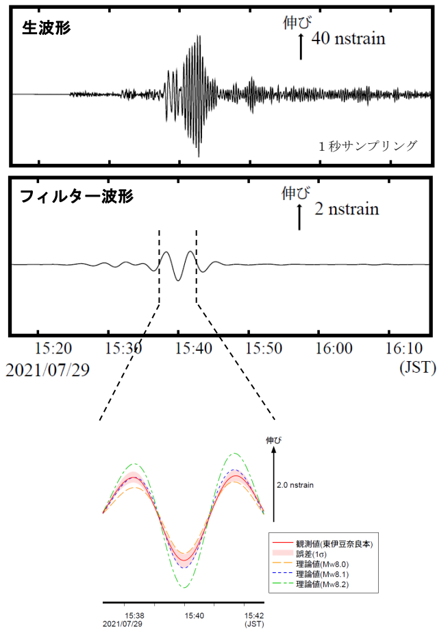
東伊豆奈良本観測点で観測された体積ひずみ波形
