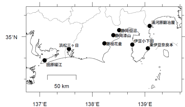
体積ひずみ計の配置図
