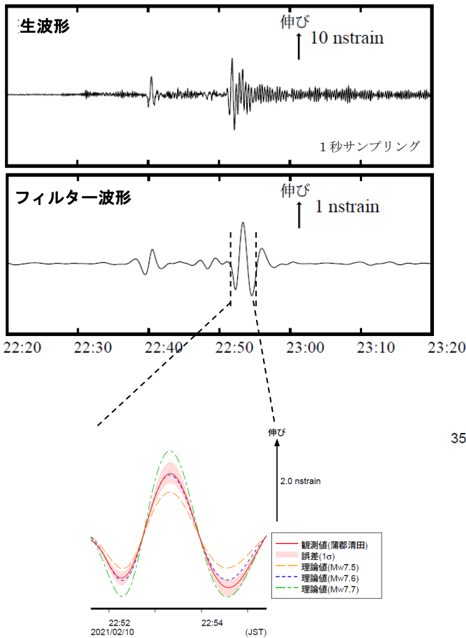
蒲郡清田観測点の観測波形と理論波形の振幅比較 (上図) データには周期 120-333 秒のバンドパスフィルタを時間軸の正逆両方向にかけている。網掛けは誤差 (1σ) の範囲を示す。
