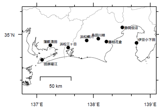
体積ひずみ計の配置図
