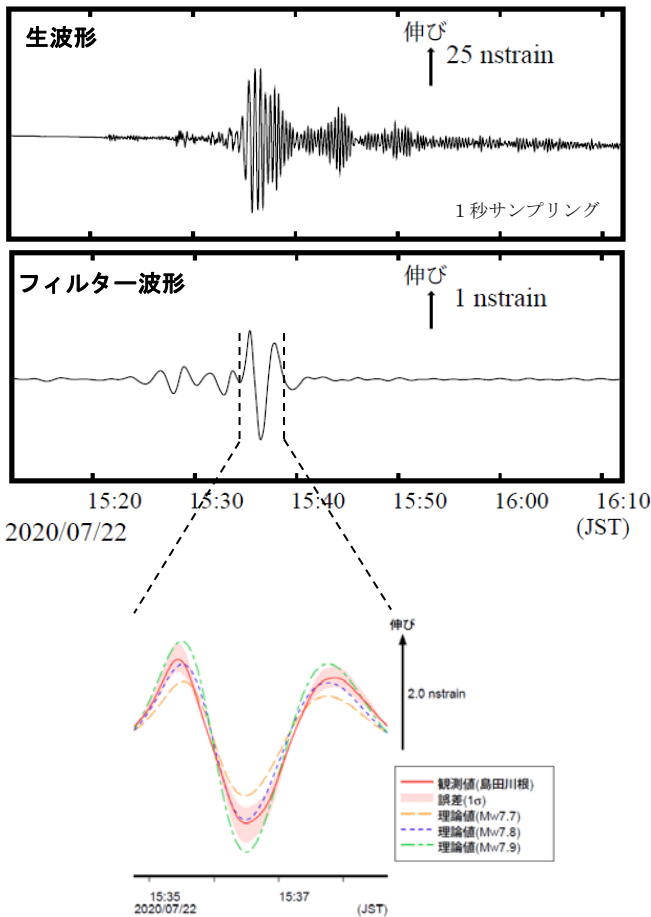
島田川根観測点の観測波形と理論波形の振幅比較（上図） データには周期 120-333 秒のバンドパスフィルタを時間軸の正逆両方向にかけている。網掛けは誤差（ 1\sigma ）の範囲を示す。
