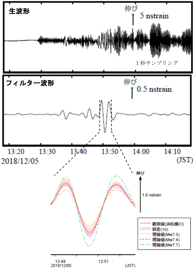
浜松横川観測点の観測波形と理論波形の振幅比較 (上図) データには周期 120-333 秒のバンドパスフィルタを時間軸の正逆両方向にかけている。網掛けは誤差 (1σ) の範囲を示す。
