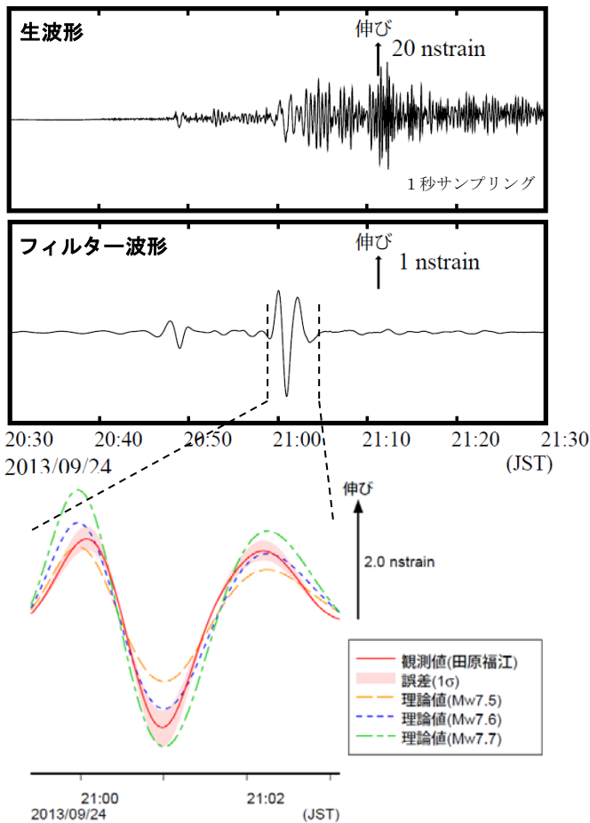
田原福江観測点の観測波形と理論波形の振幅比較（上図） データには周期 120-333 秒のバンドパスフィルタを時間軸の正逆両方向にかけている。網掛けは誤差（1 \sigma ）の範囲を示す。
