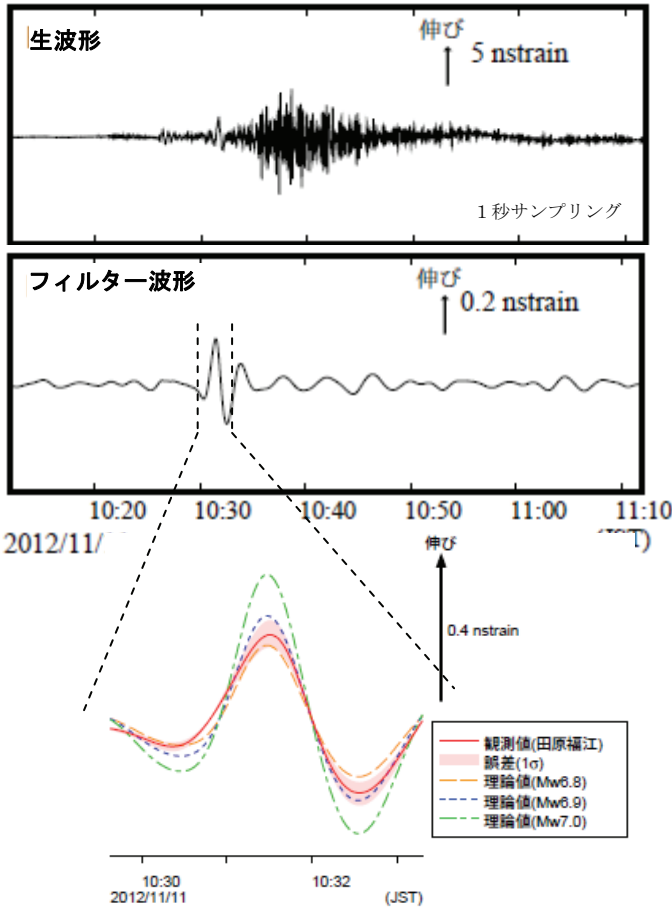
田原福江観測点の観測波形と理論波形の振幅比較（上図） データには周期 120-333 秒のバンドパスフィルタを時間軸の正逆両方向にかけている。網掛けは誤差 ( 1\sigma ) の範囲を示す。
