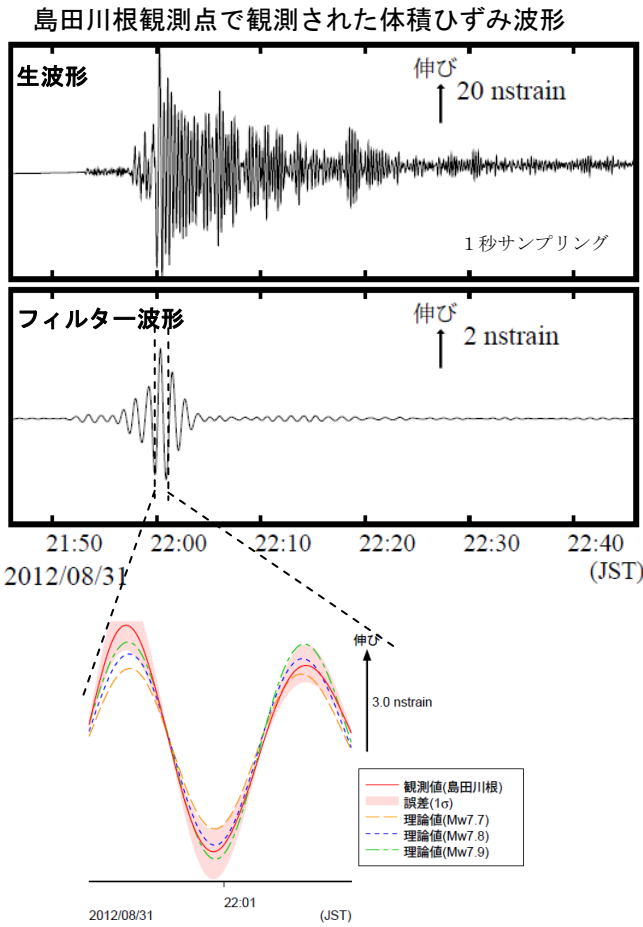
島田川根観測点の観測波形と理論波形の振幅比較 (上図) データには周期 60～90 秒のバンドパスフィルタを時間軸の正逆両方向にかけている。網掛けは誤差 (1σ) の範囲を示す。
