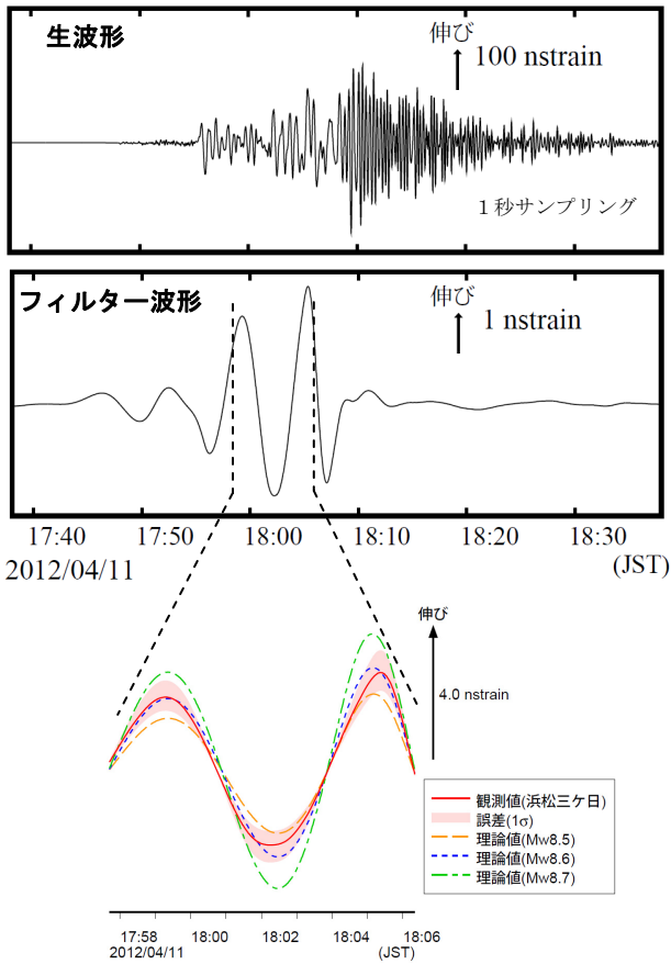
浜松三ヶ日観測点で観測された体積ひずみ波形
