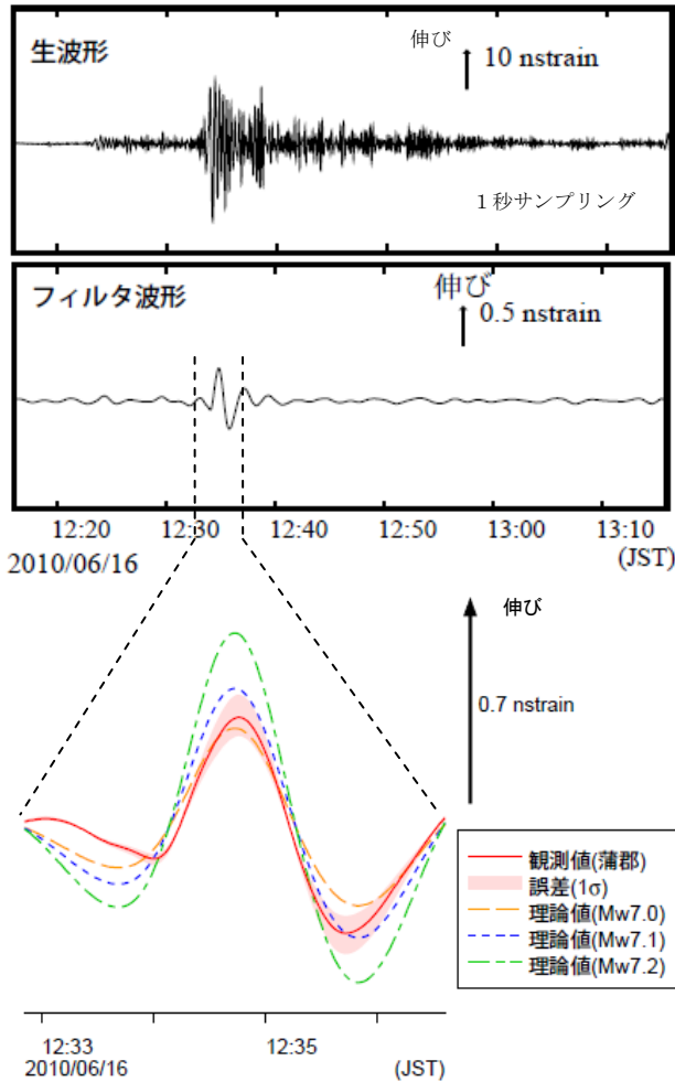
蒲郡観測点の観測波形と理論波形の振幅比較 (上図) データには周期 120~333 秒のバンドパスフィルタを時間軸の正逆両方向にかけている。網掛けは誤差 (1σ) の範囲を示す。
