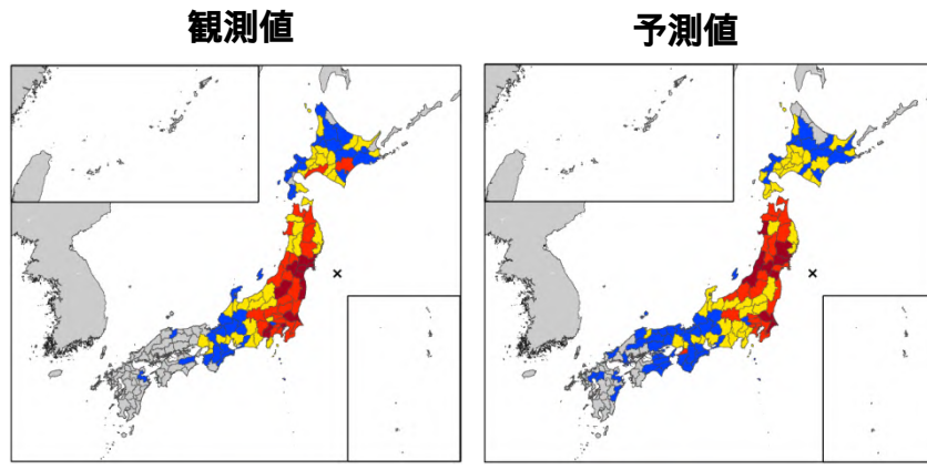
図A-6 東北地方太平洋沖地震（Mj8.4）における長周期地震動階級の予測結果
