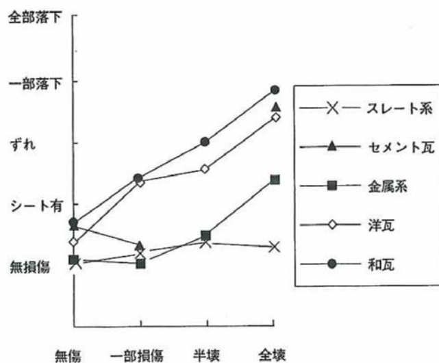
図 6.1.9 構造被害と屋根材被害の関係：全地域木造
