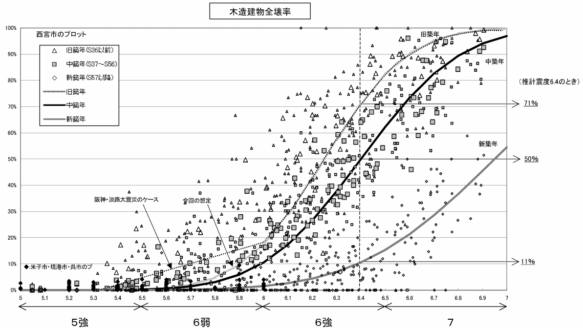
図1 中央防災会議（2005）による木造建物全壊率と計測震度の関係
