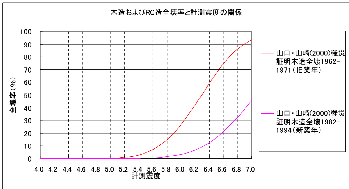
図2 山口・山崎（2000）による木造建物全壊率と計測震度の関係
