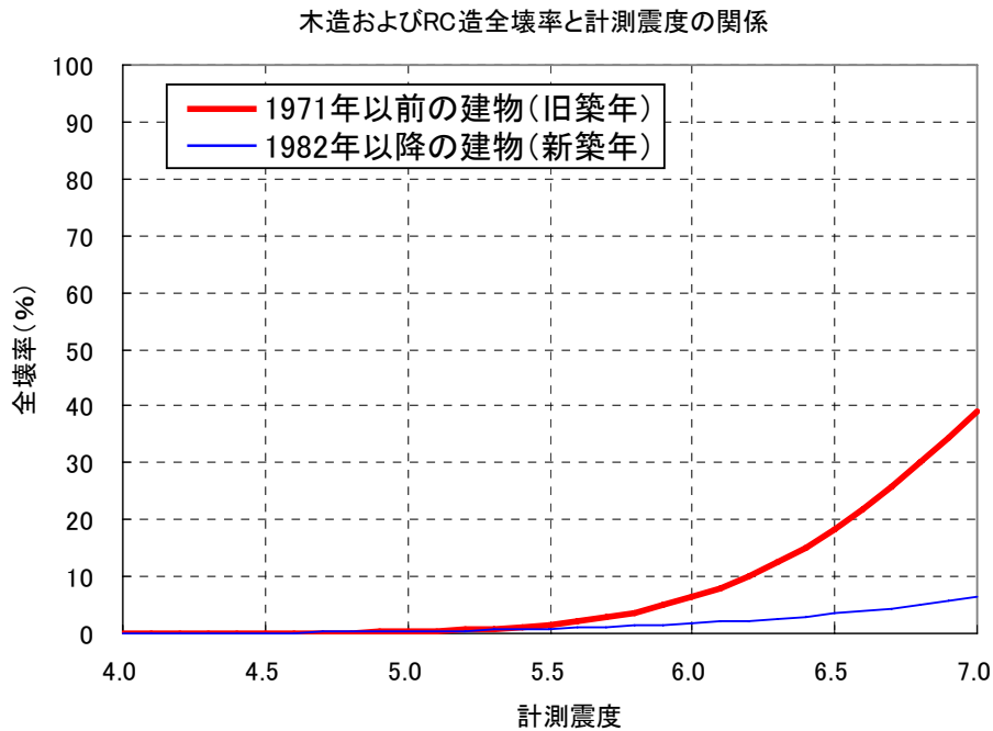
図2 山口・山崎(2000)による鉄筋コンクリート建物の全壊率と計測震度の関係
