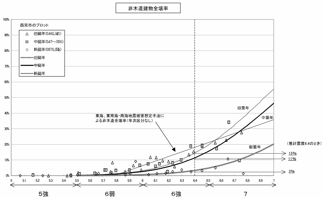
図 5 中央防災会議（2005）による非木造建築の全壊率と計測震度の関係
