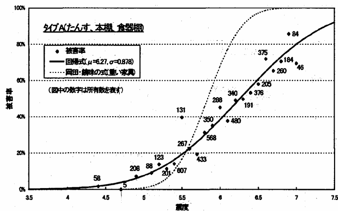
図10 家財被害関数(タイプAの場合)
