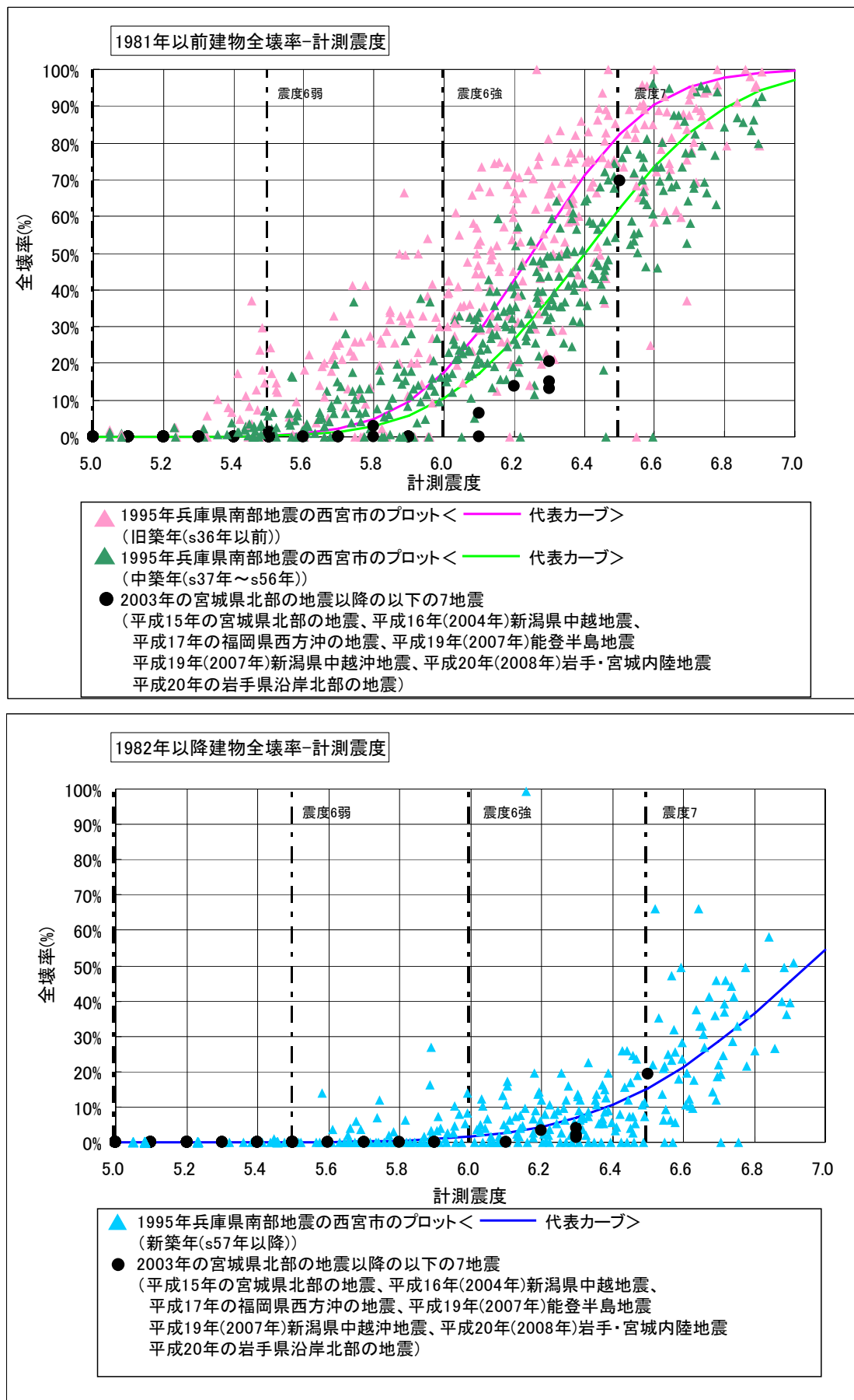
図 5-2 木造全壊率と計測震度の関係 兵庫県南部地震の木造被害との重ね合わせ (中央防災会議のデータ 16 に加筆)
