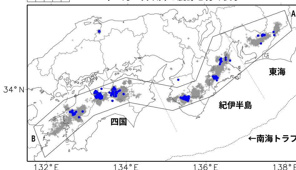
震央分布図（2022年09月15日～2023年09月14日：過去1年間、M全て、深さ全て） 2023年09月08日以降の震源を青く表示
