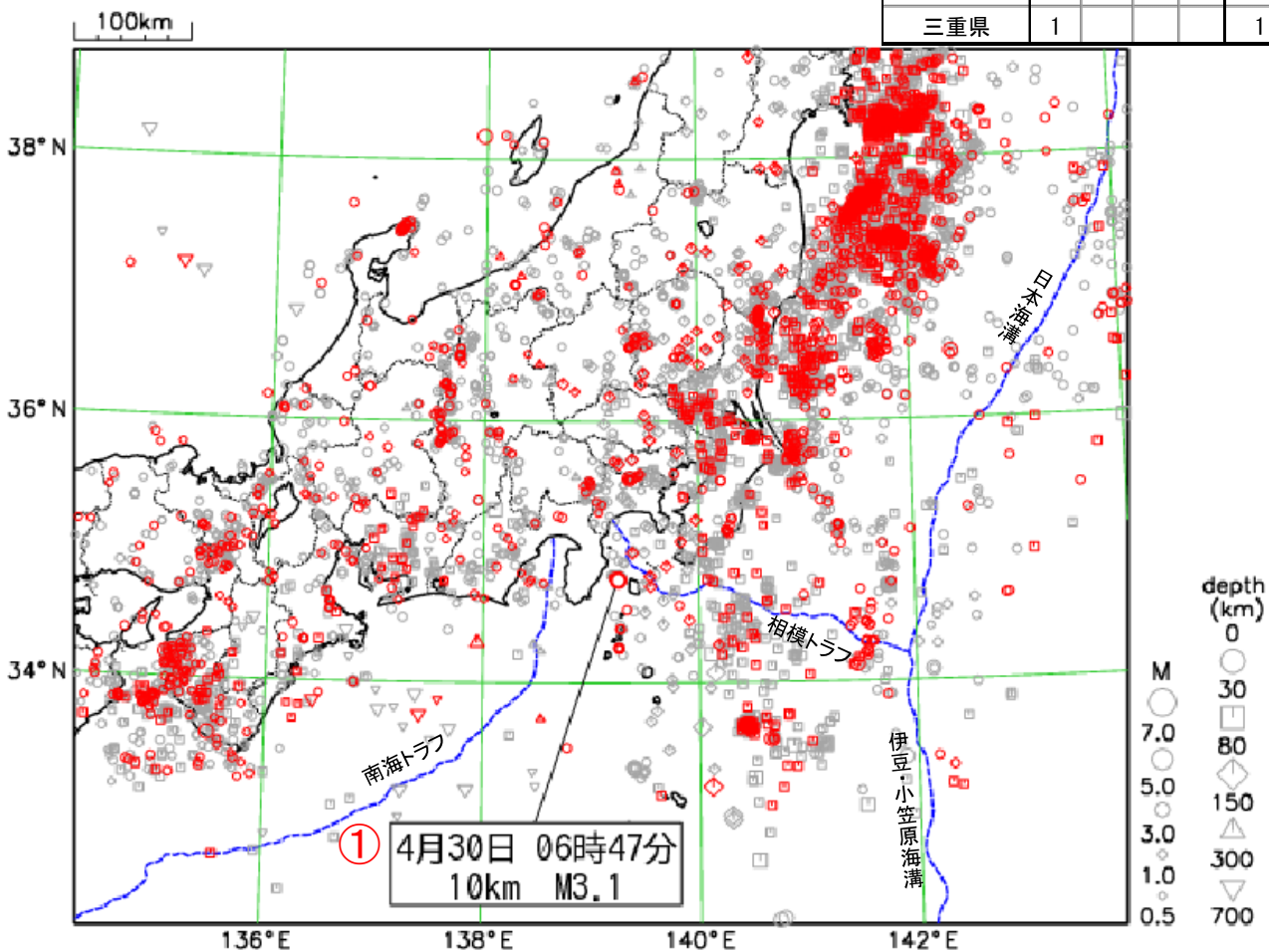
震央分布図
