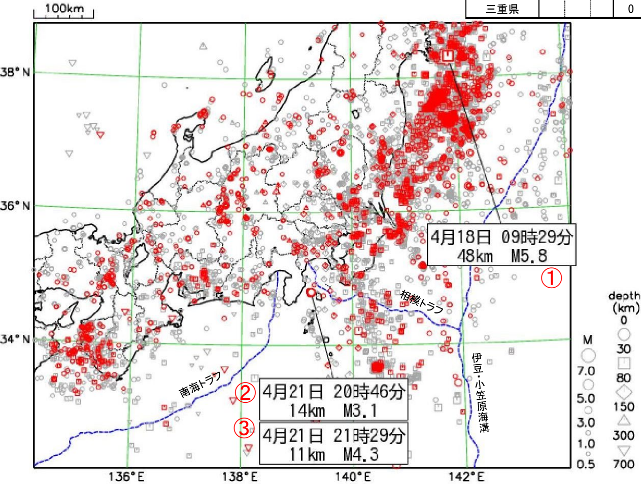
震央分布図
