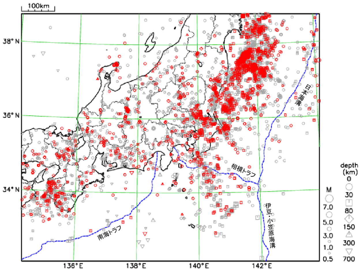
震央分布図
