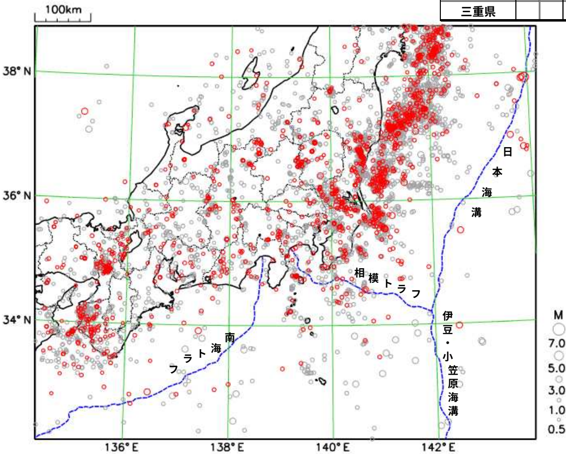
震央分布図 (2018 年 7 月 10 日 00 時 00 分～2018 年 8 月 9 日 24 時 00 分、深さ 0～400 km、M \geq 0.5 の地震) *2018 年 8 月 3 日以降に発生した地震の震央を赤で表示しています。
